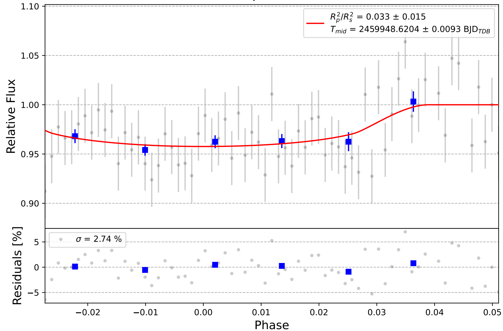
Qatar-4 b
