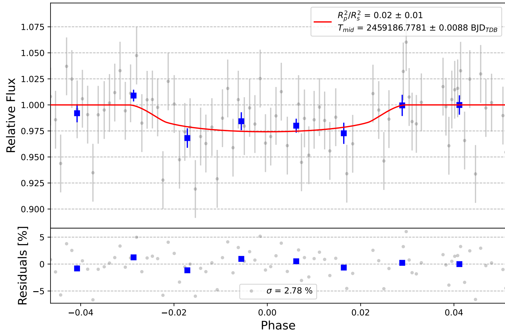
Qatar-4 b
