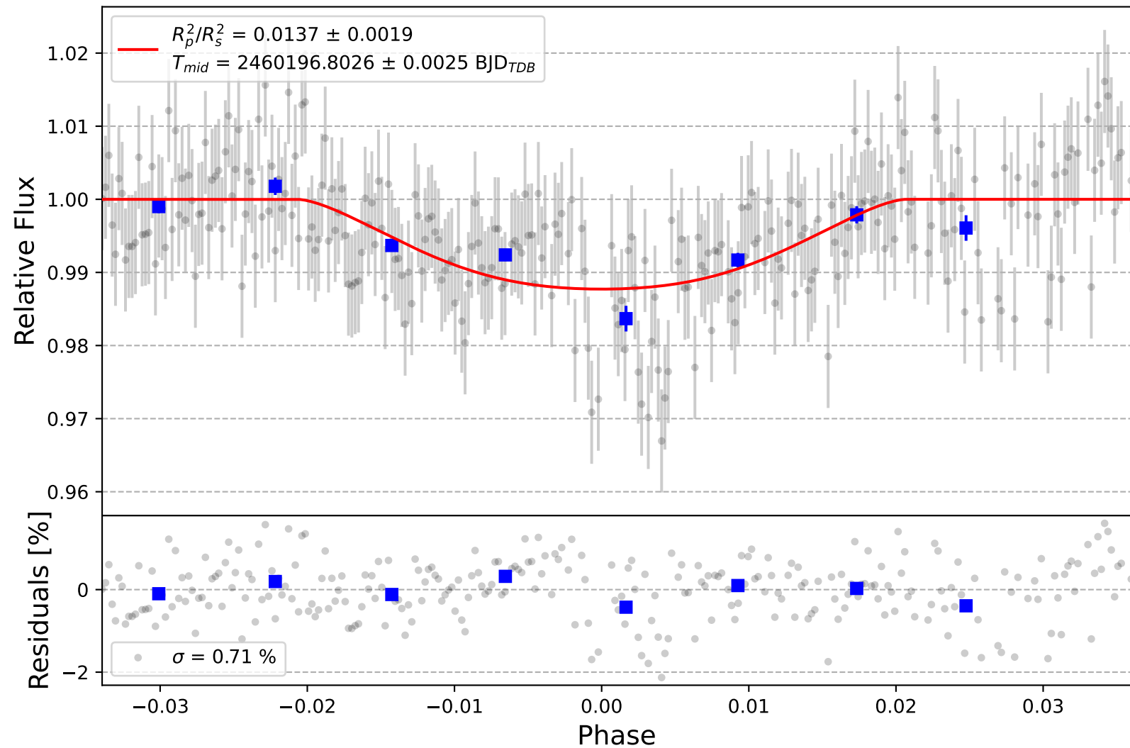
TOI-1431 b
