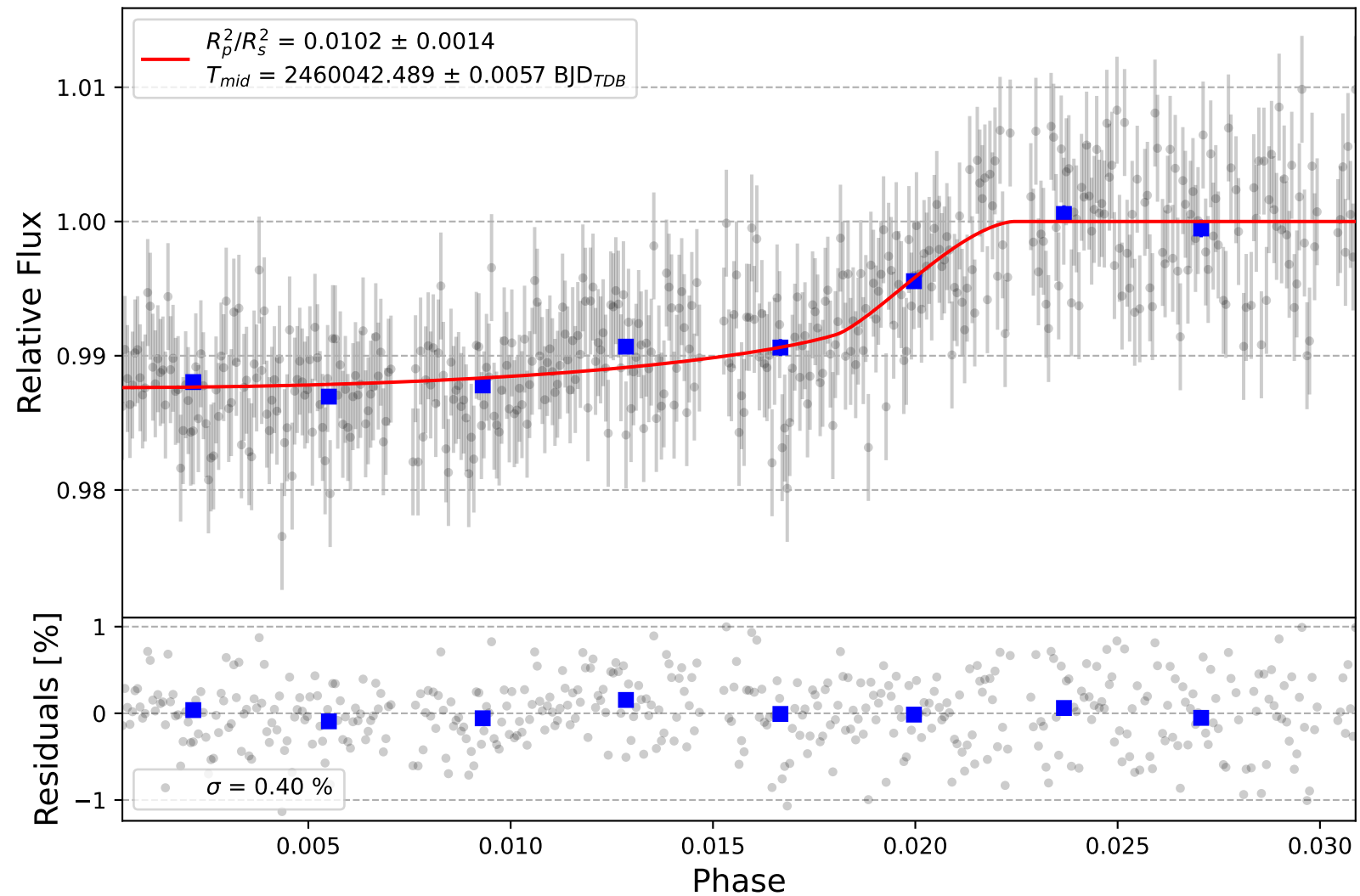
TOI-150.01
