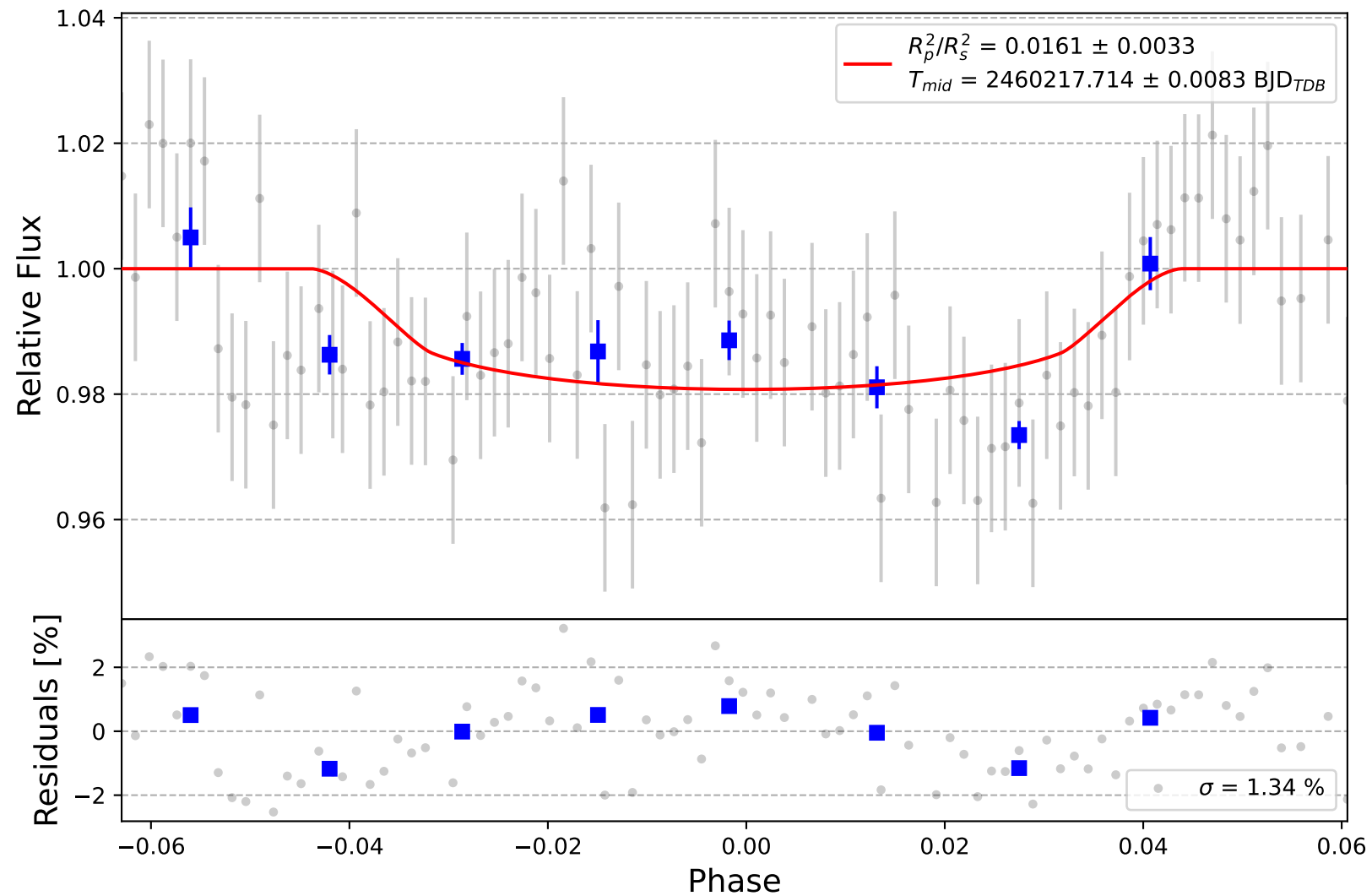
TOI-2046 b
