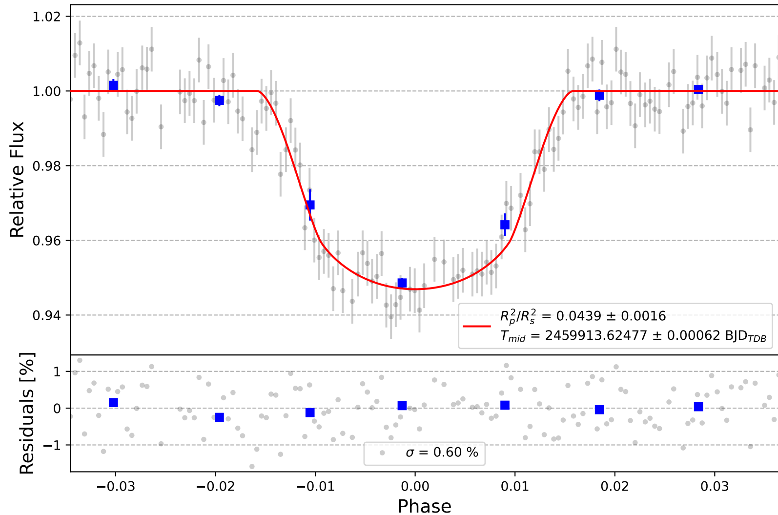
TOI-3714 b
