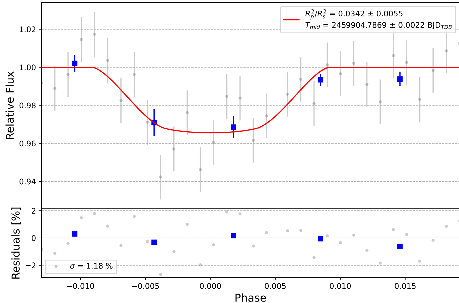
TOI-3757 b
