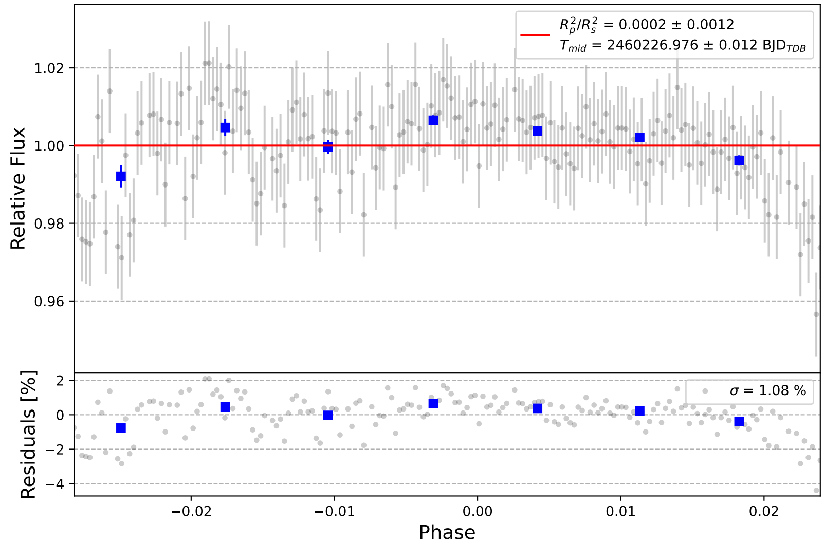
TOI-3807 b
