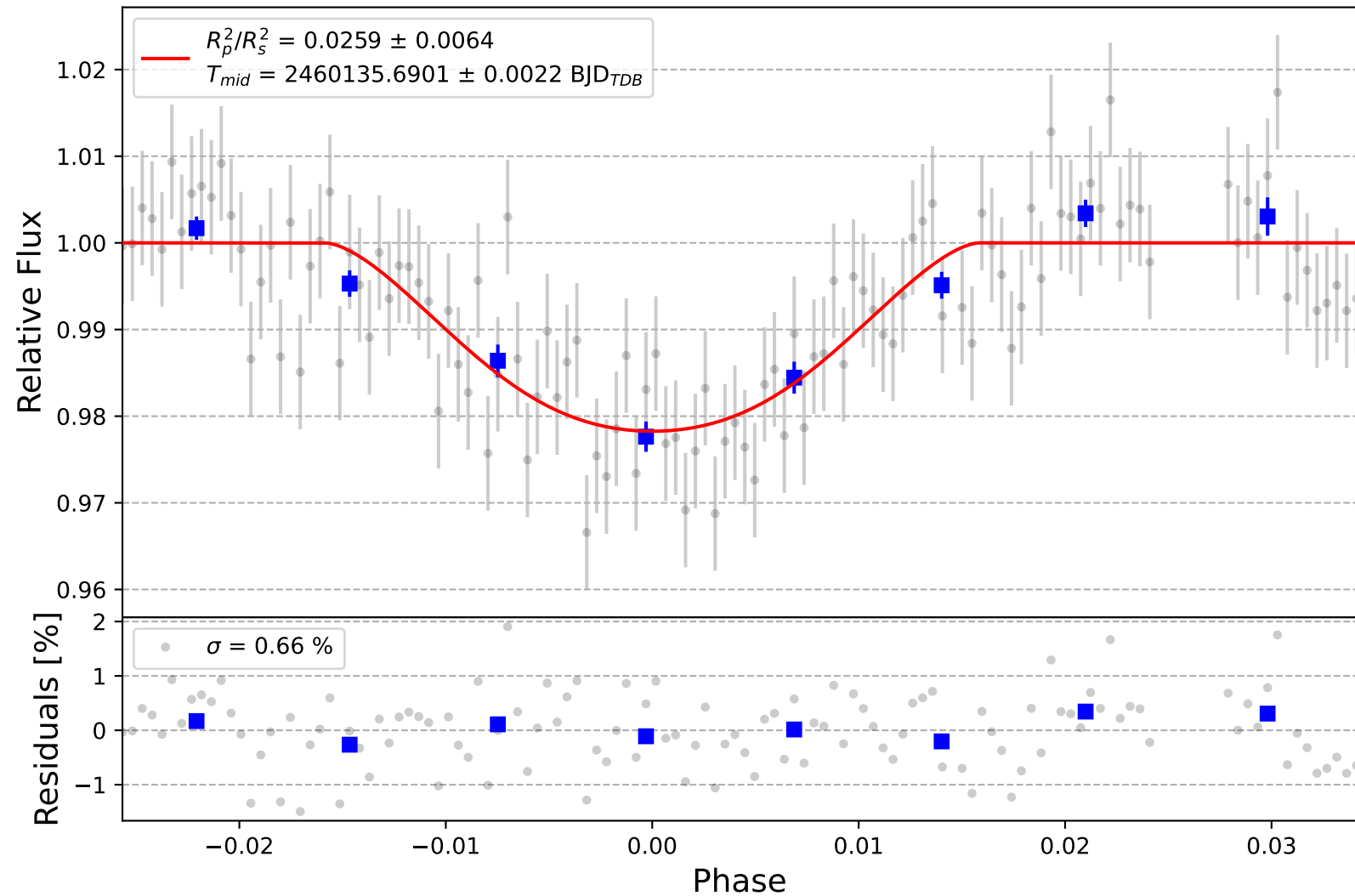
TOI-4463 A b
