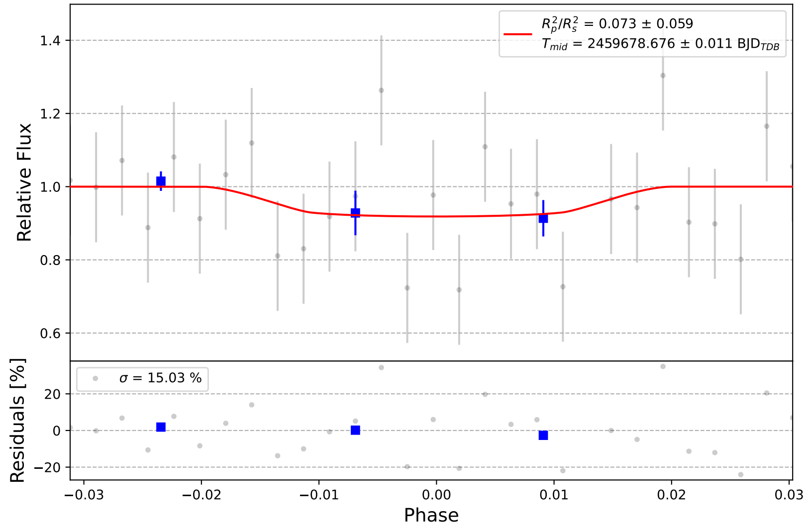
TOI-519 b
