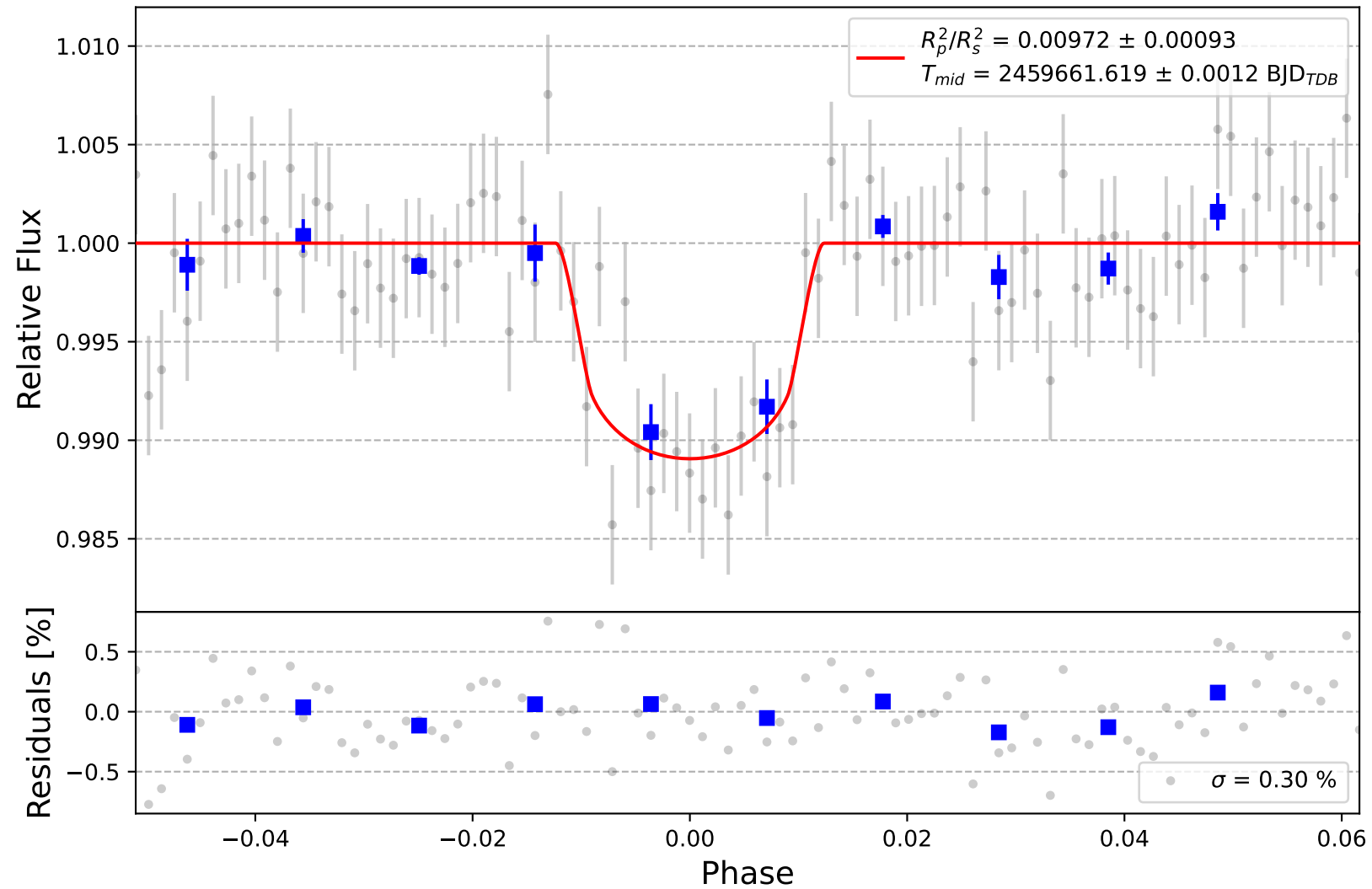
TOI-674 b
