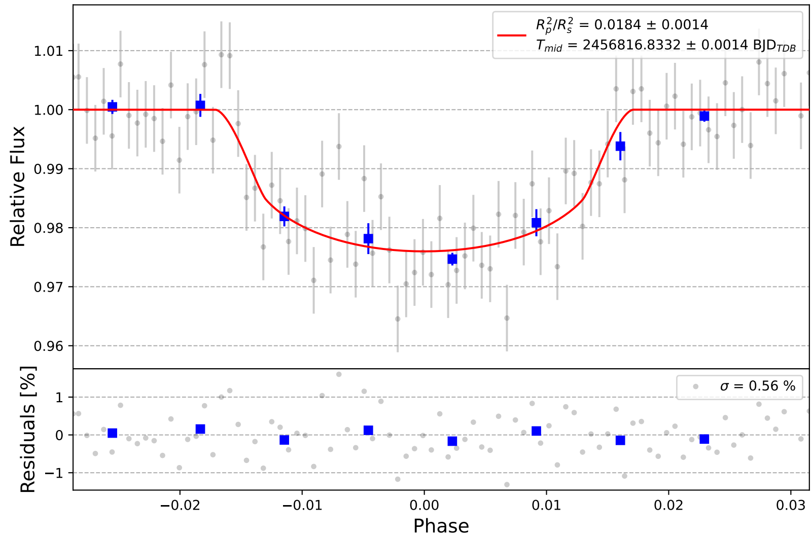
TrES-1 b
