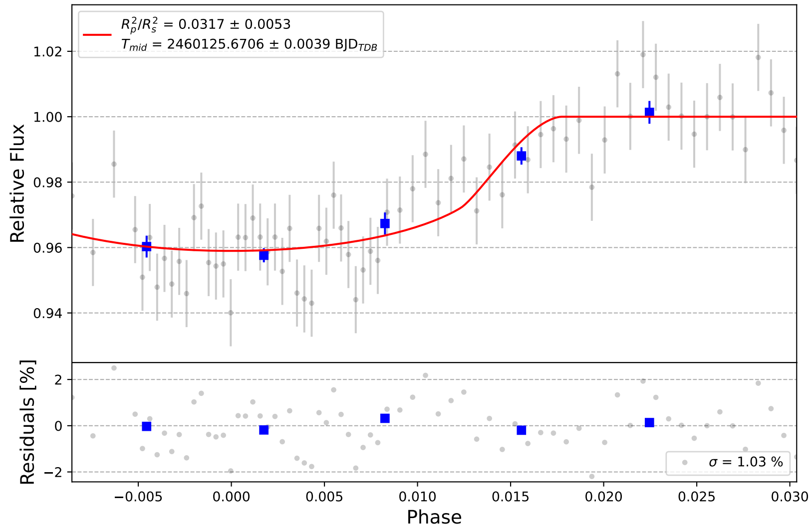
TrES-1 b
