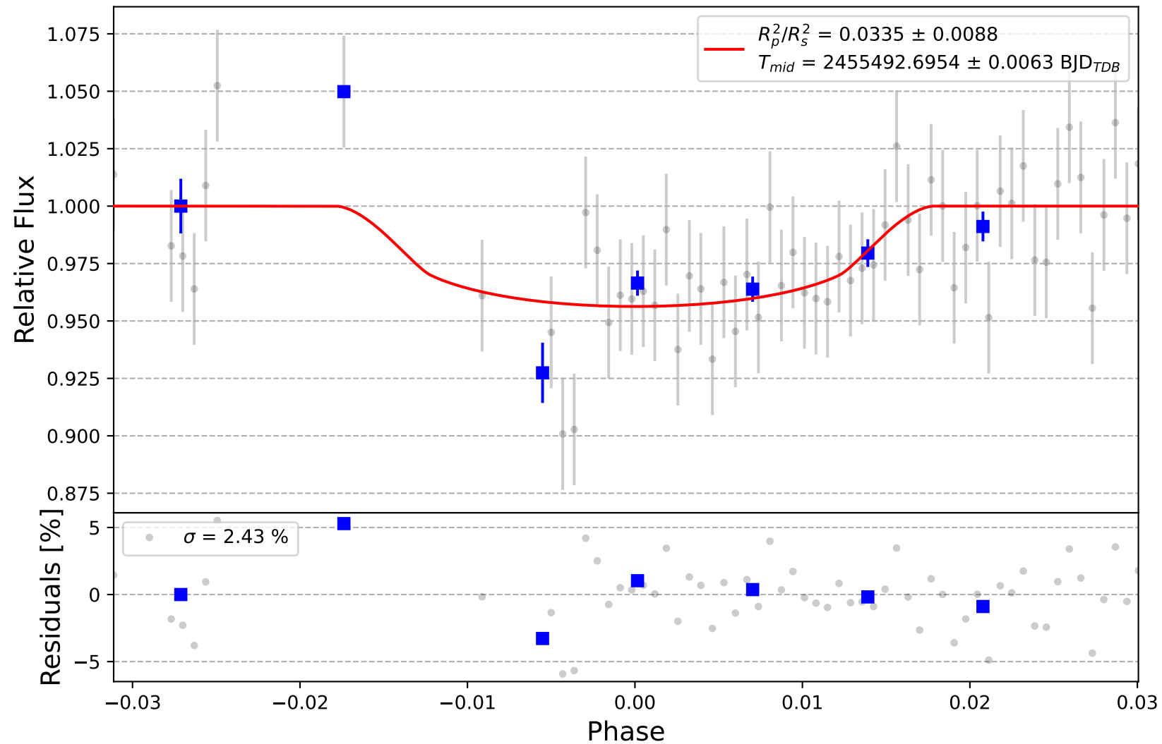
TrES-1 b
