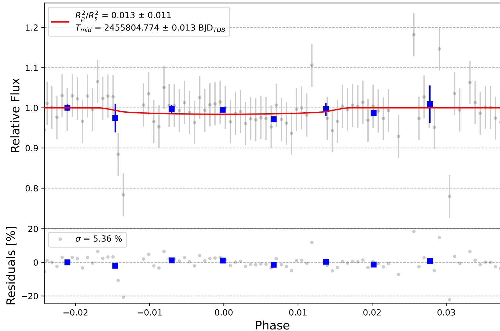
TrES-1 b
