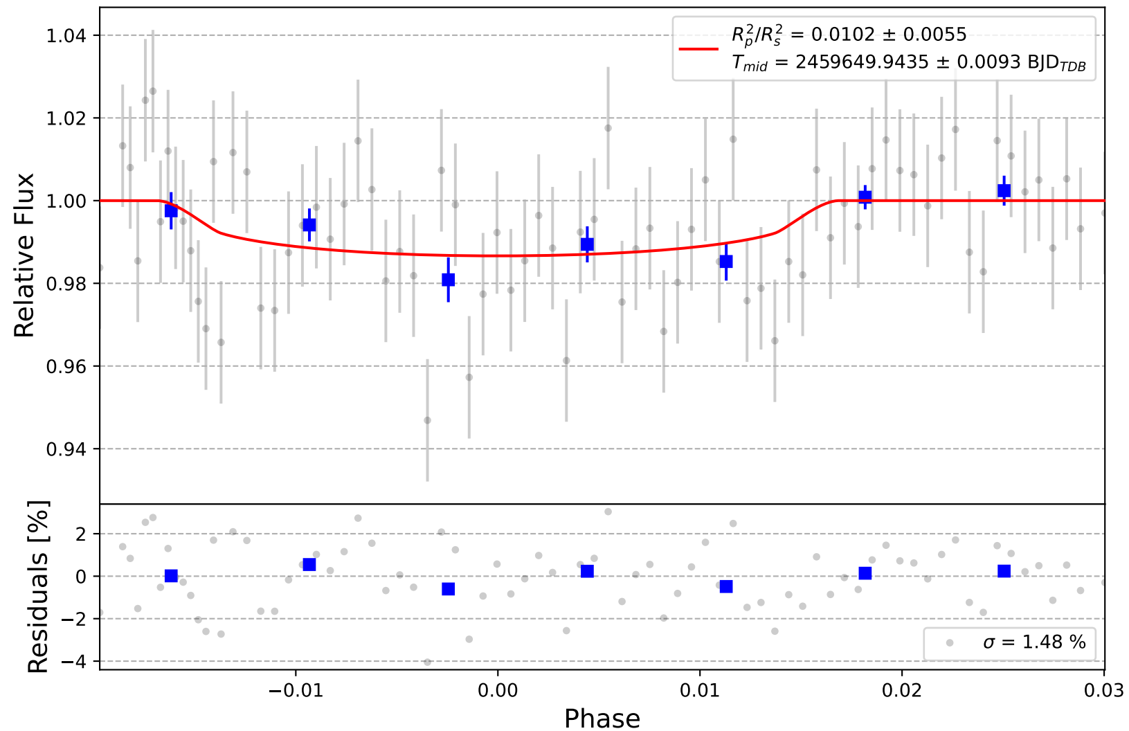
TrES-1 b
