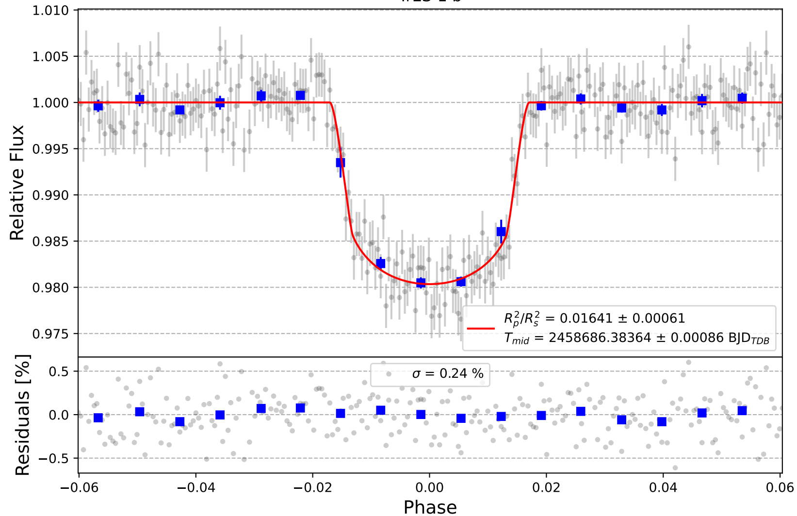
TrES-1 b
