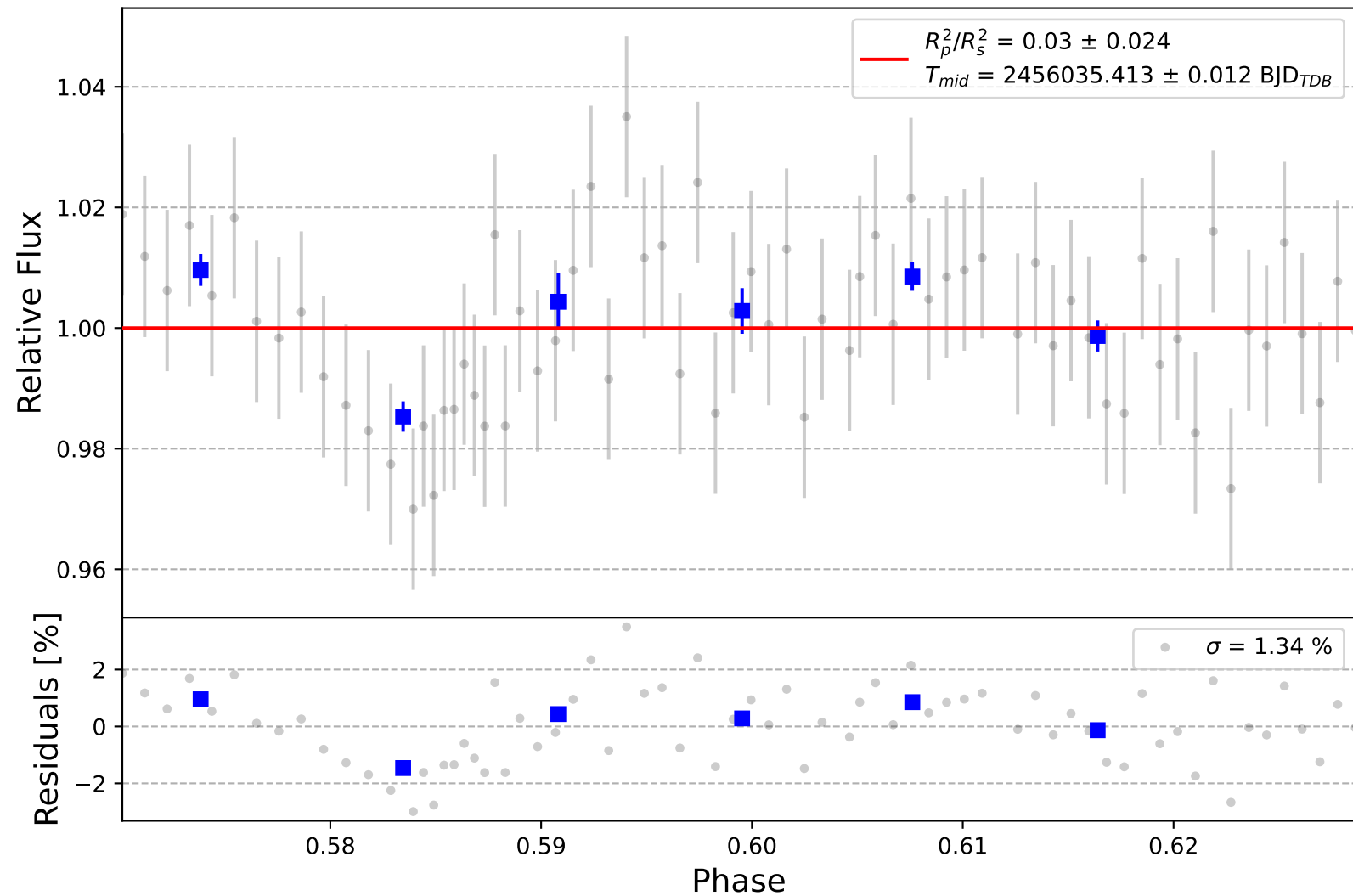
TrES-2 b
