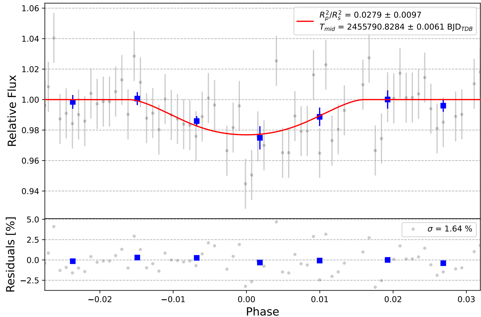
TrES-2 b
