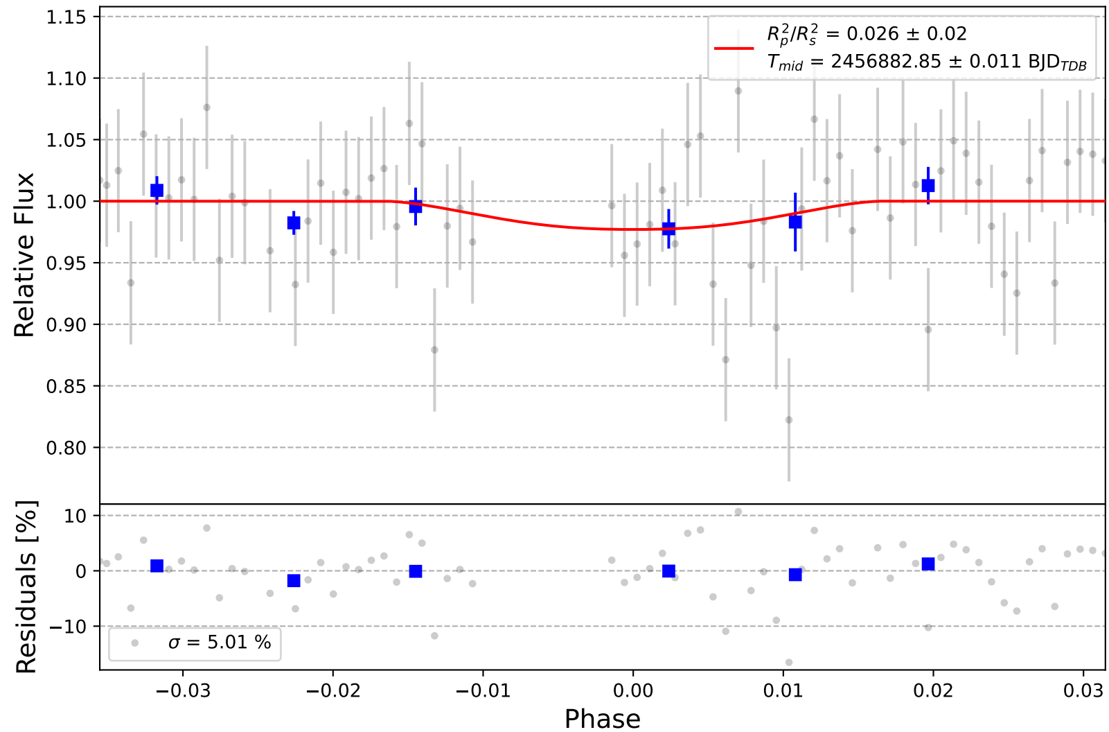
TrES-2 b
