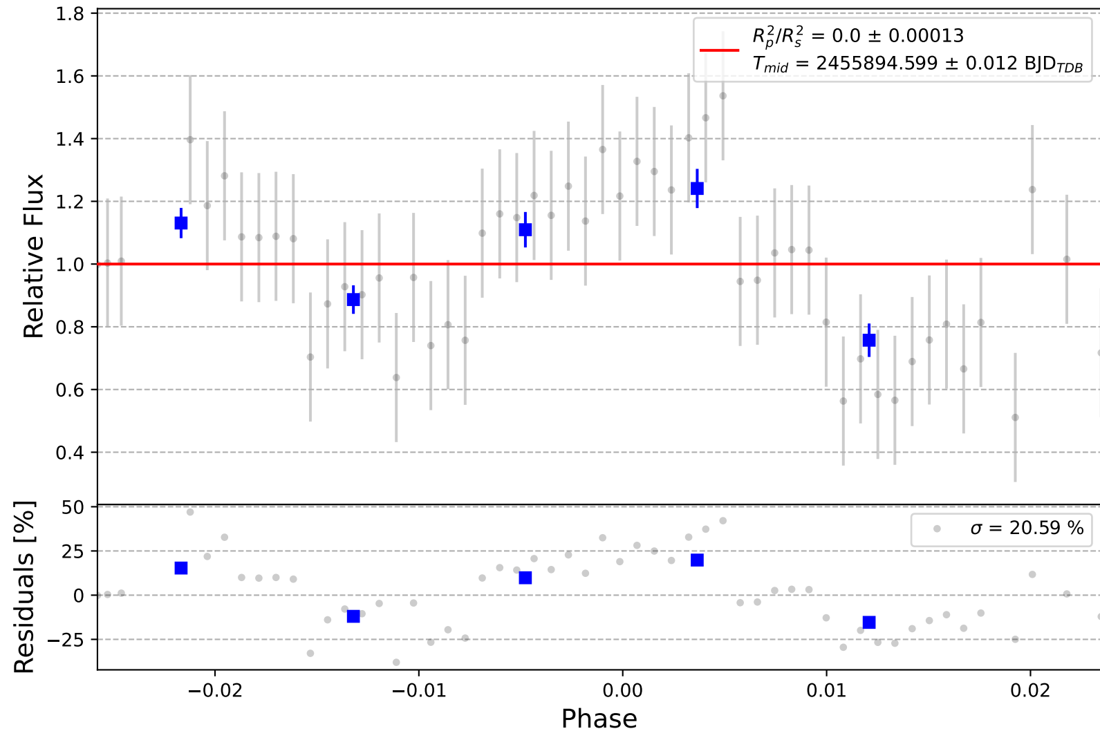
TrES-2 b
