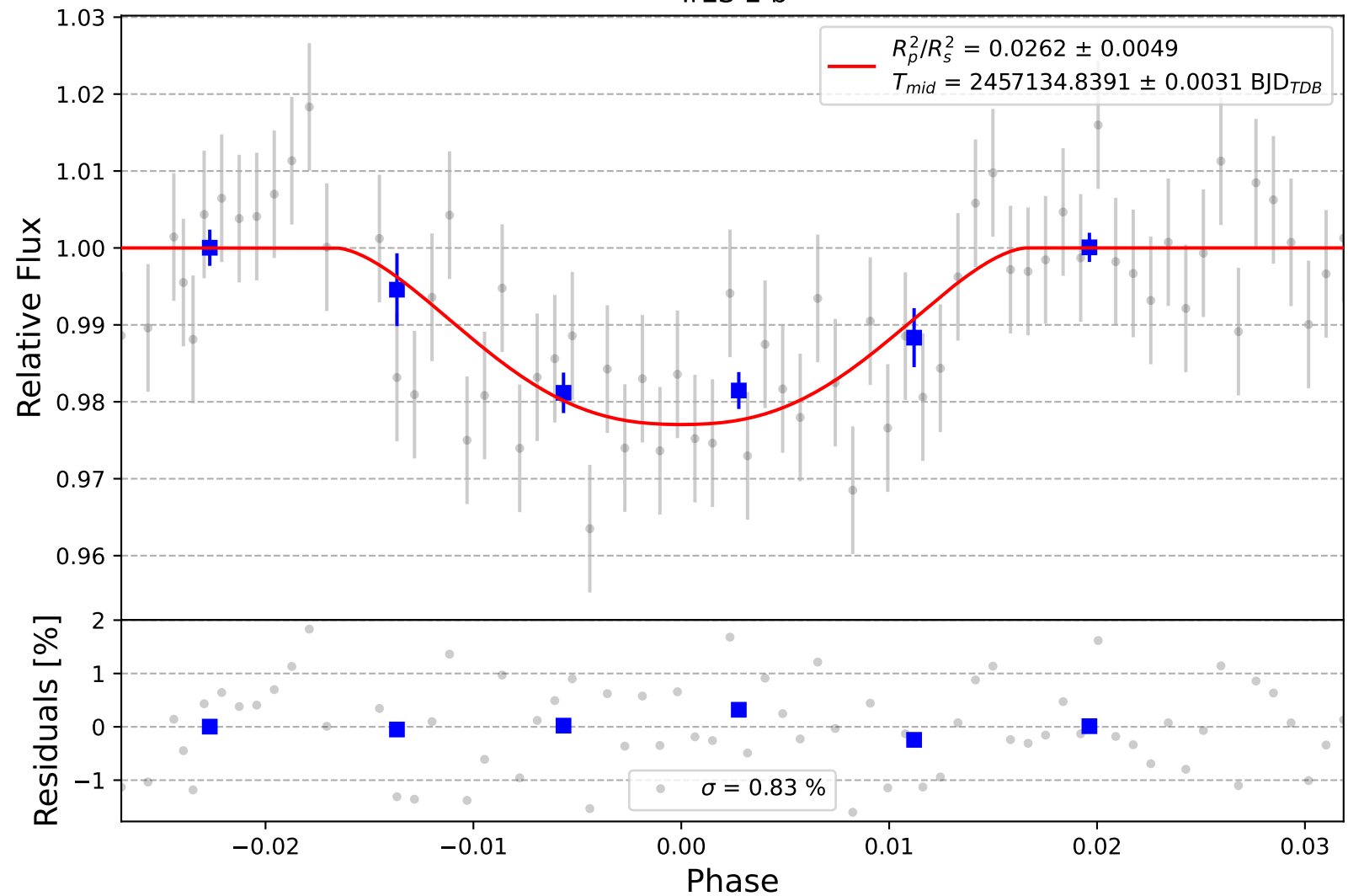
TrES-2 b
