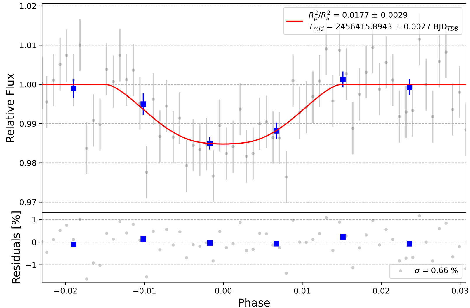
TrES-2 b
