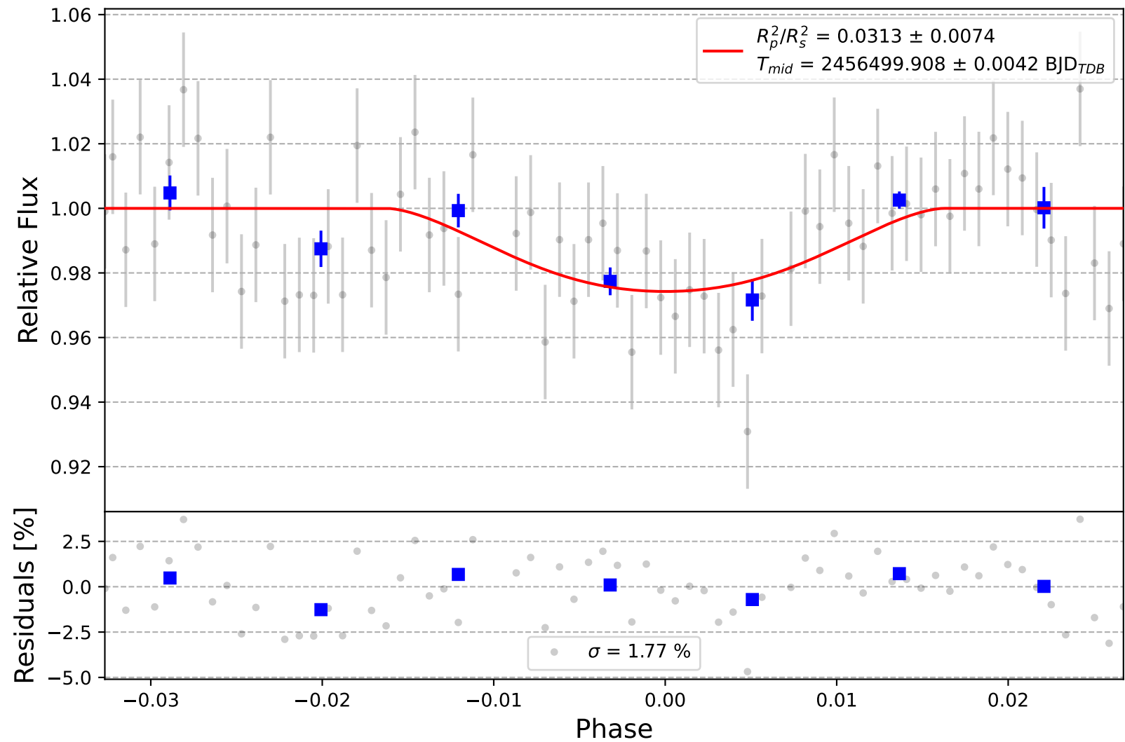
TrES-2 b
