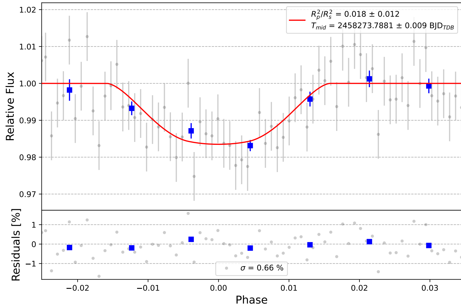
TrES-2 b
