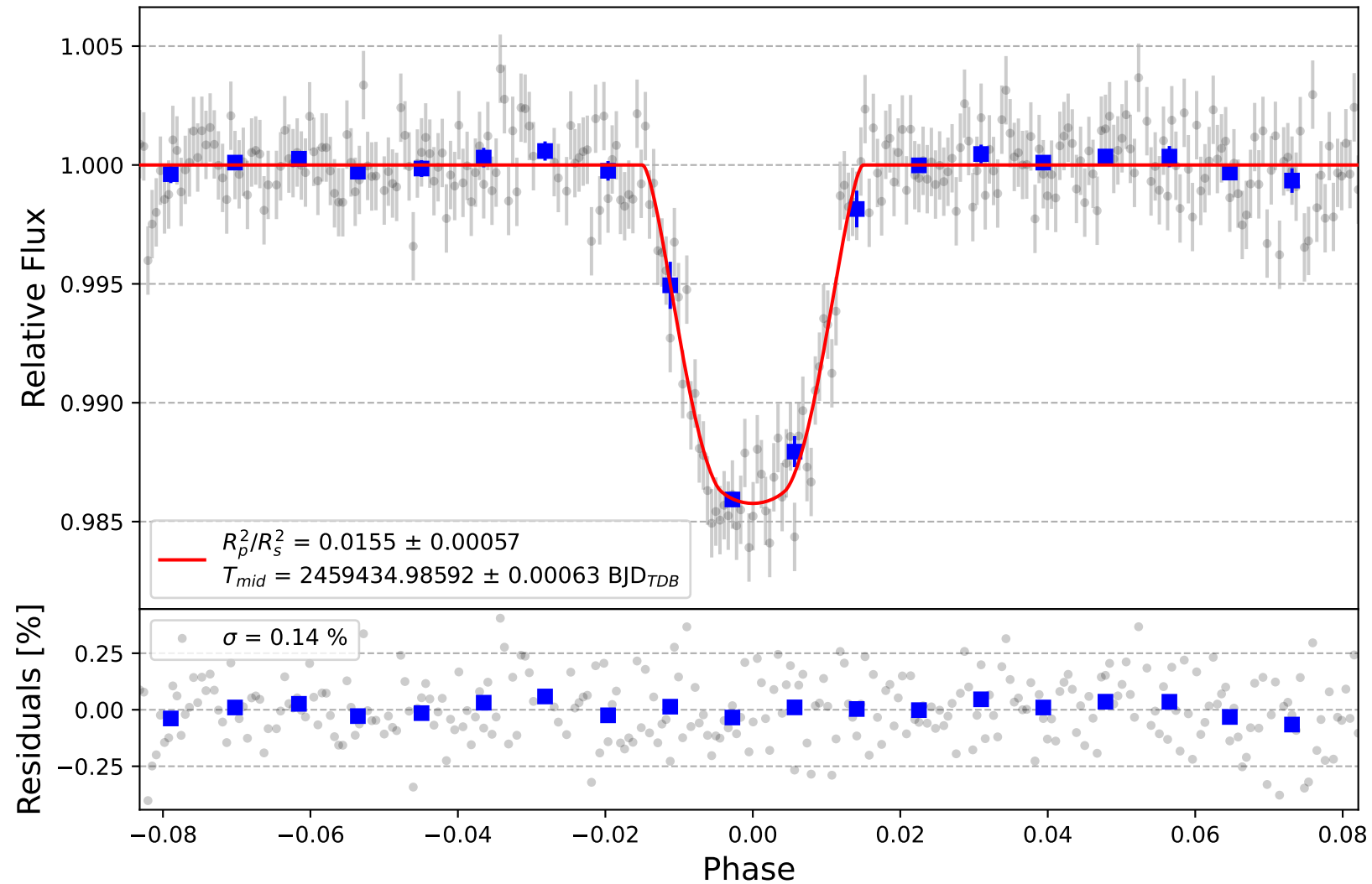
TrES-2 b
