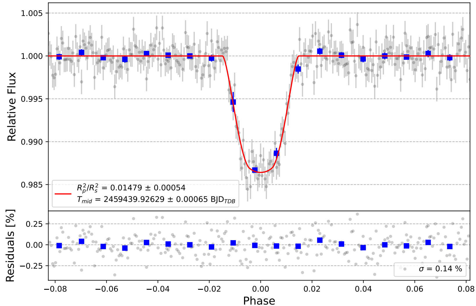
TrES-2 b
