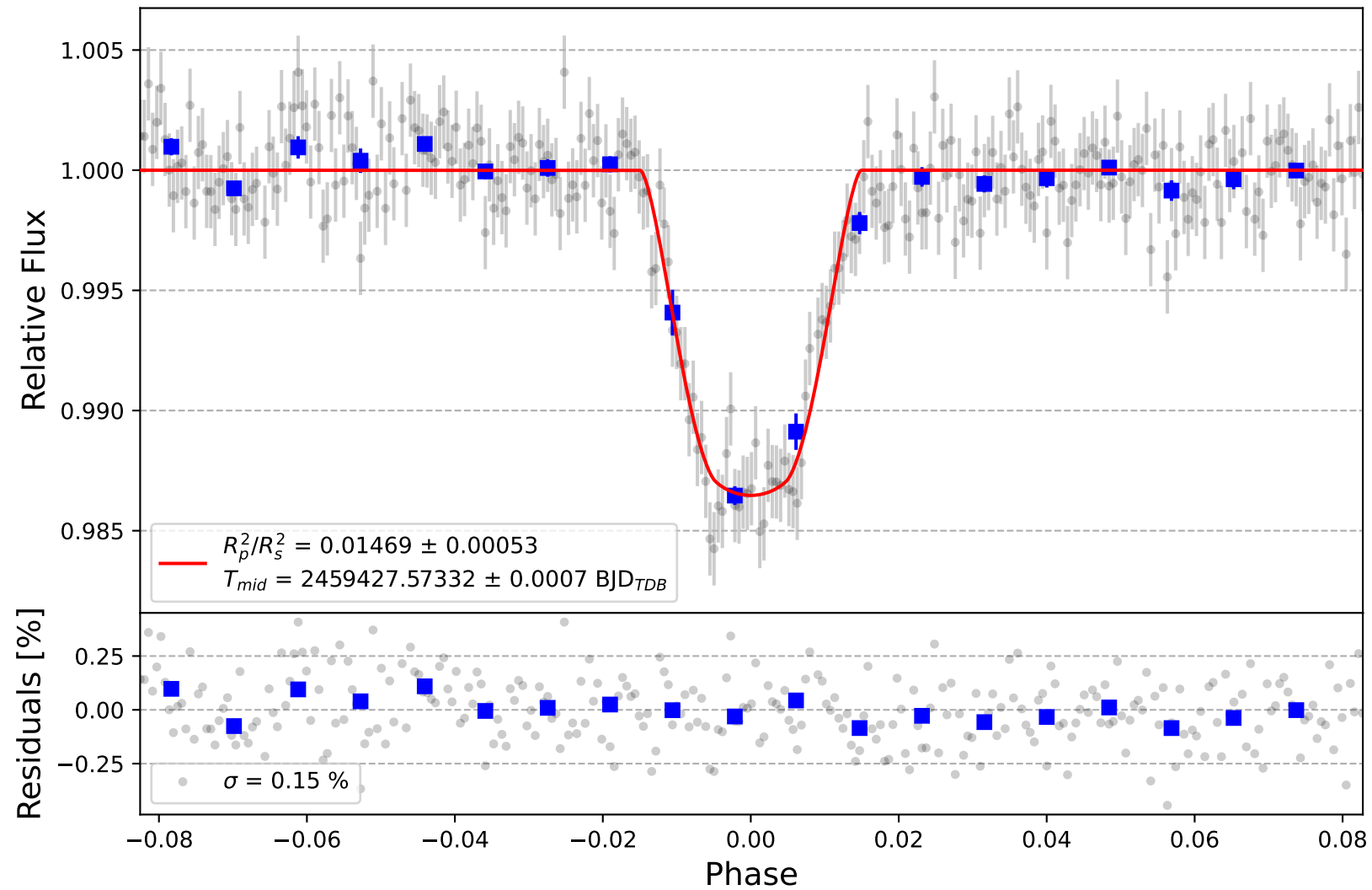
TrES-2 b
