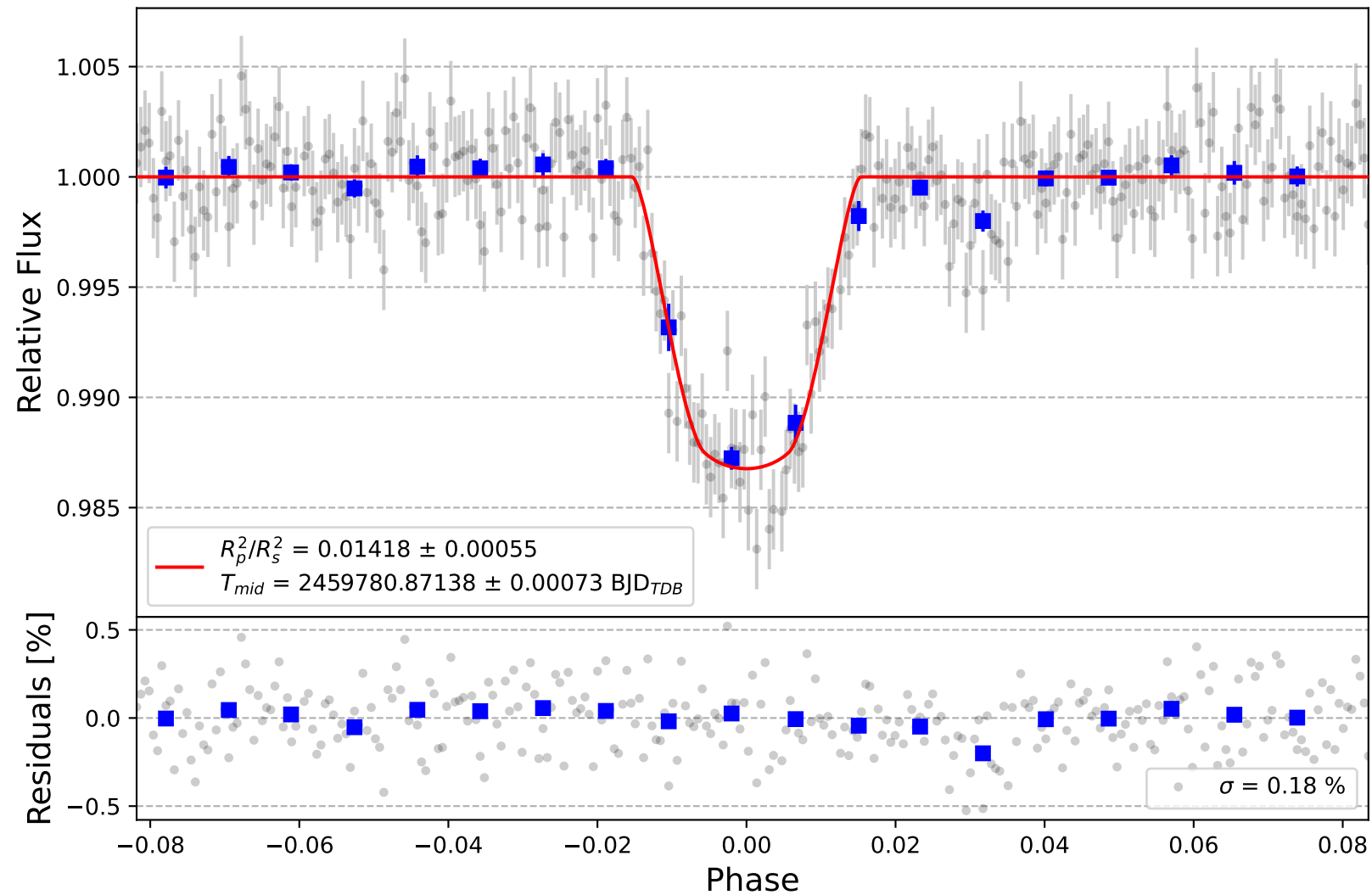
TrES-2 b
