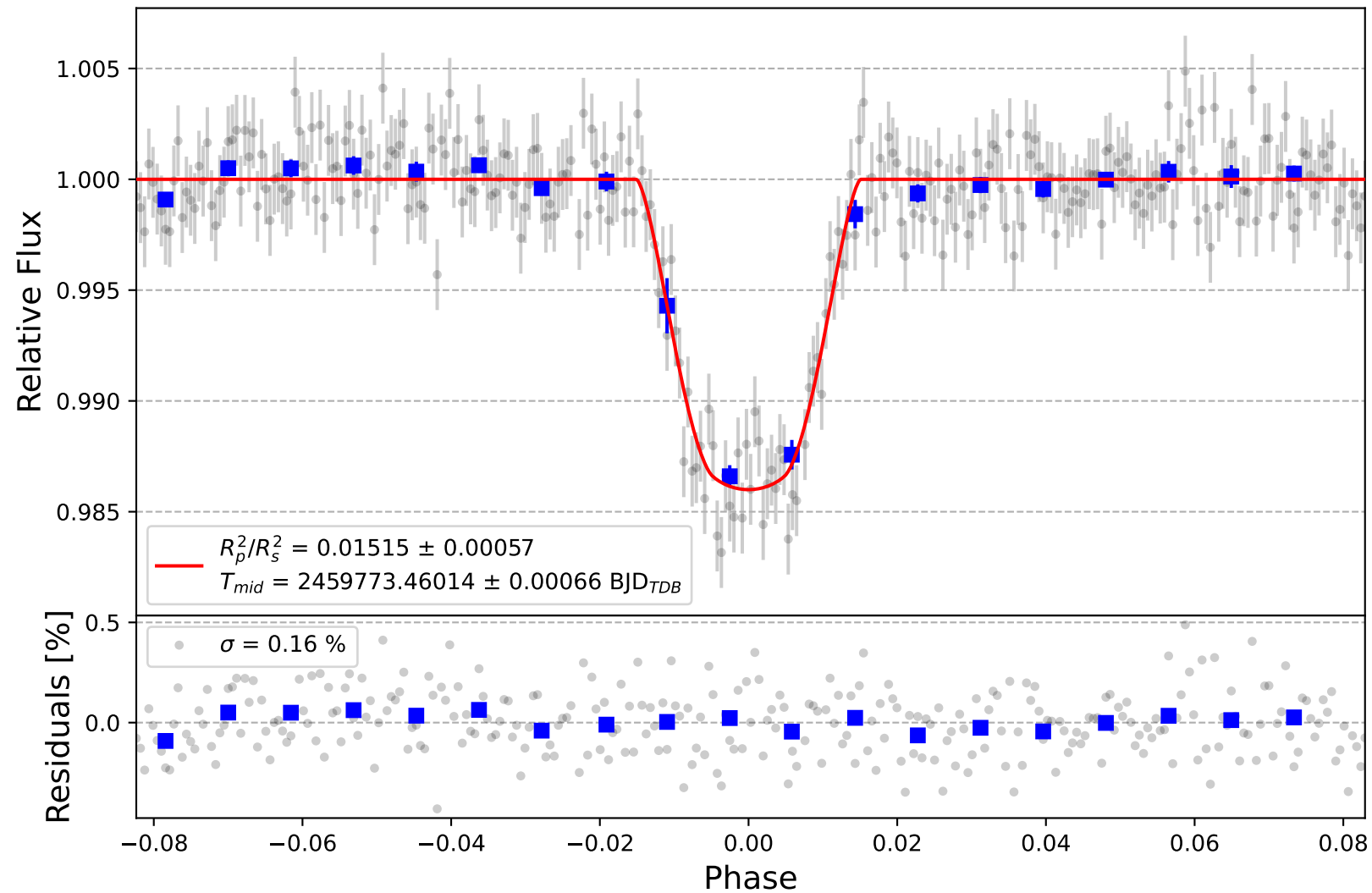
TrES-2 b
