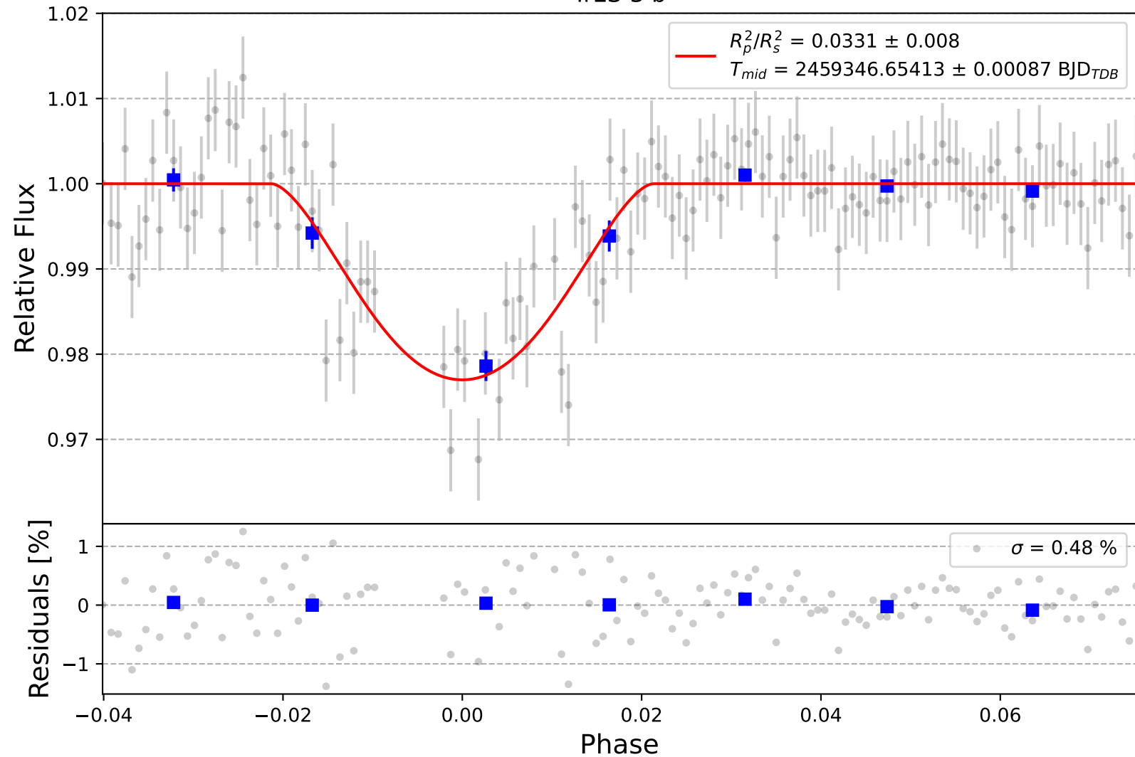
TrES-3 b
