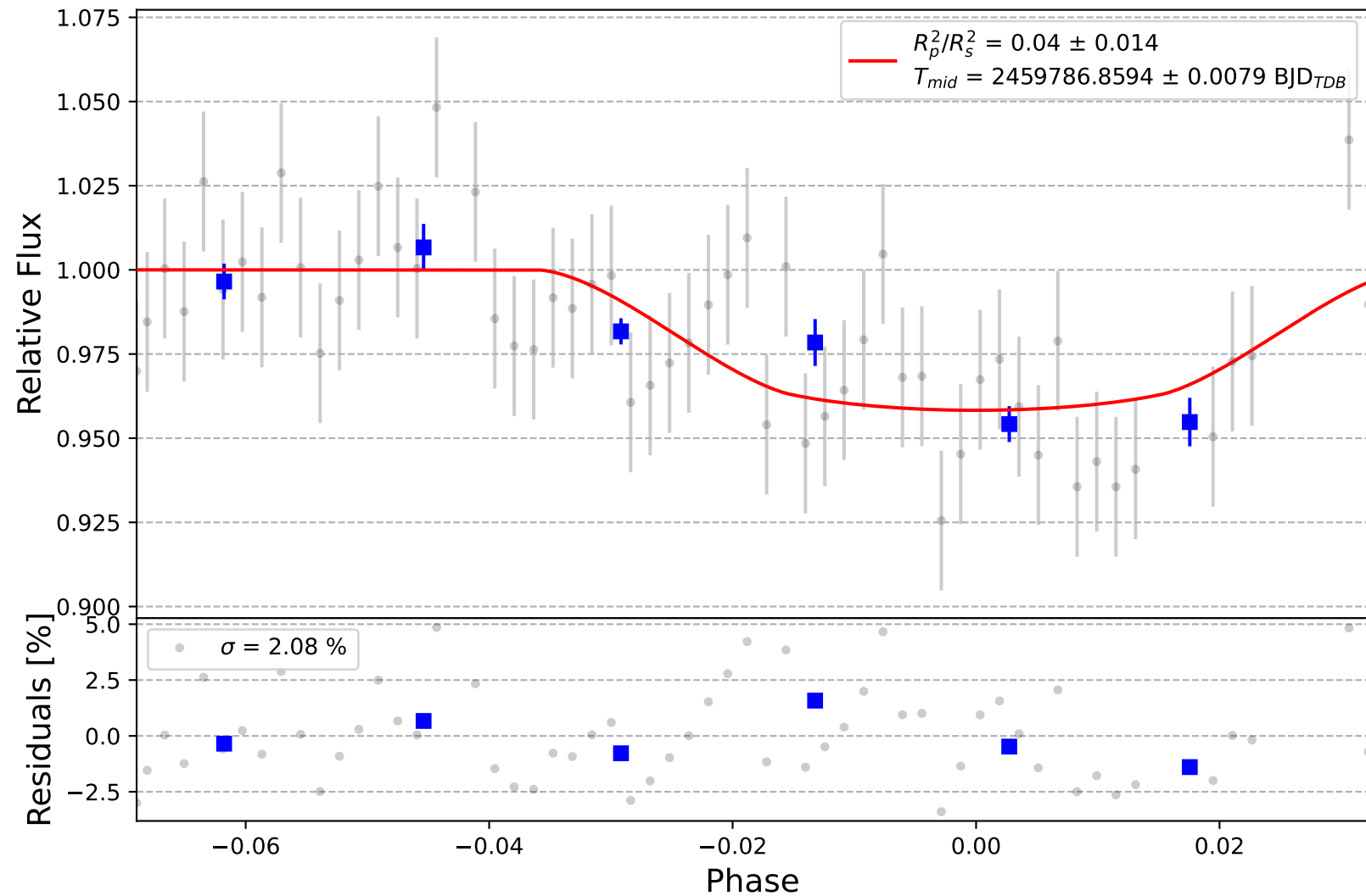
TrES-3 b
