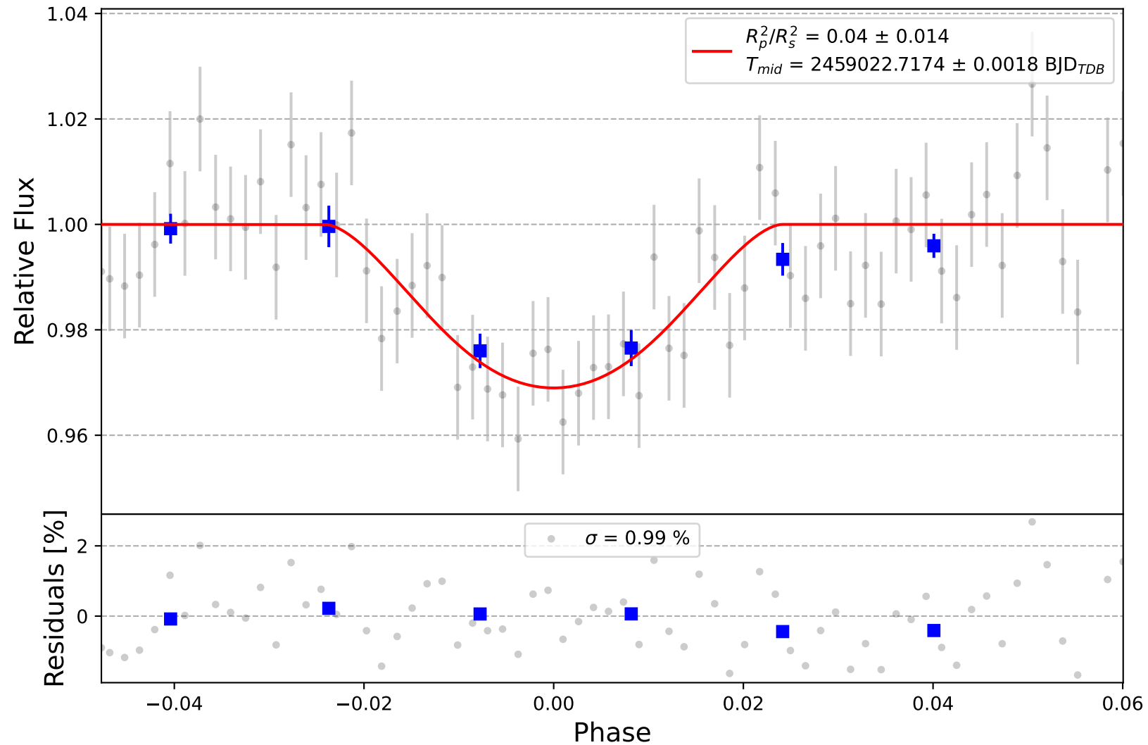
TrES-3 b
