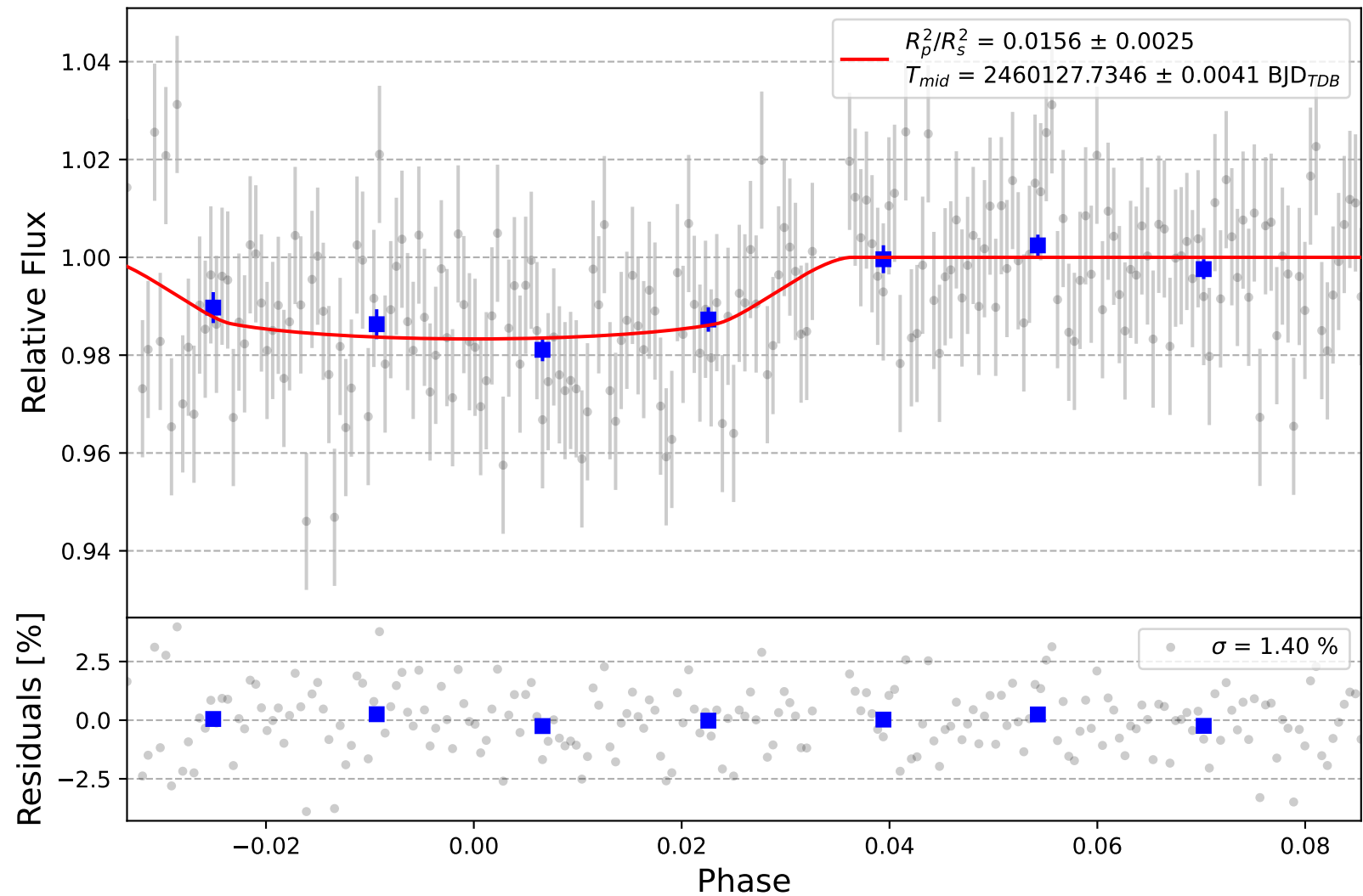
TrES-3 b
