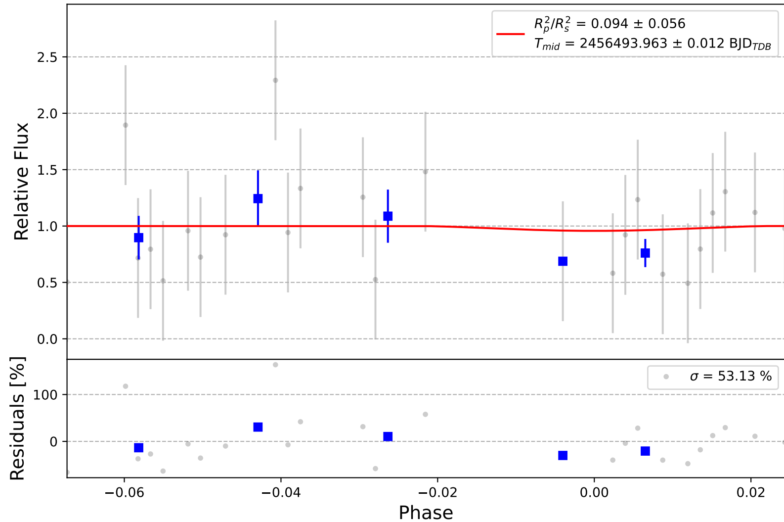
TrES-3 b
