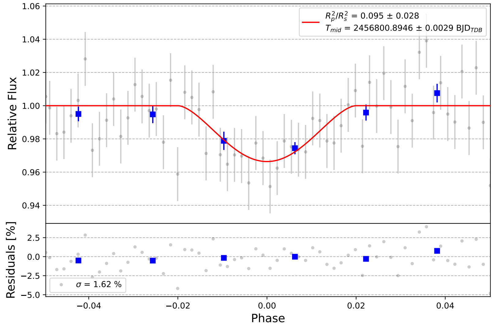
TrES-3 b
