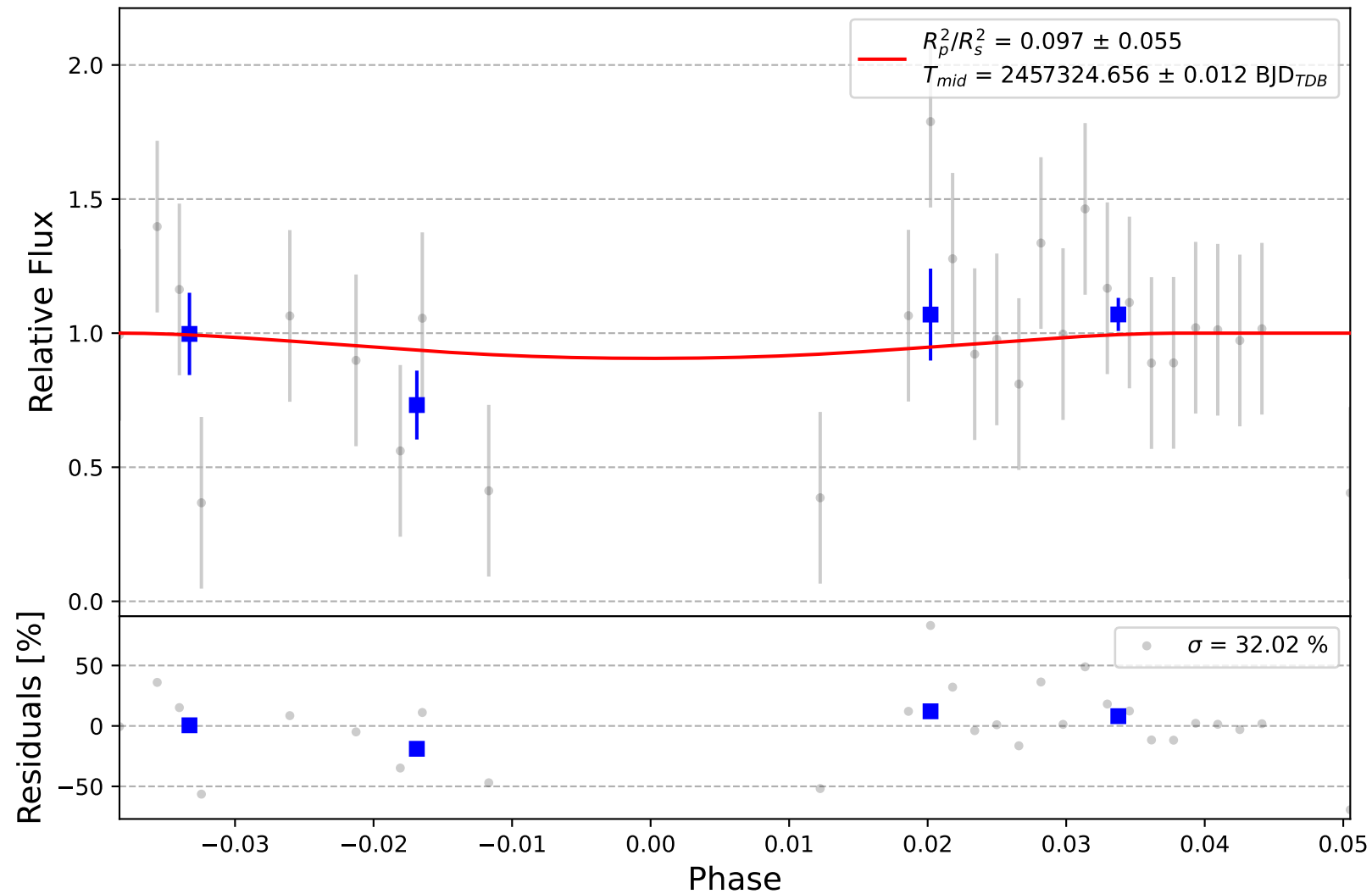
TrES-3 b
