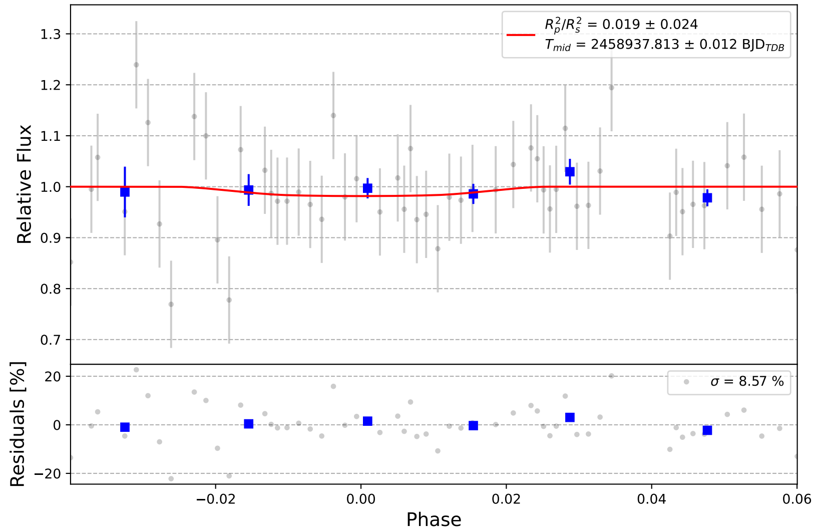
TrES-3 b
