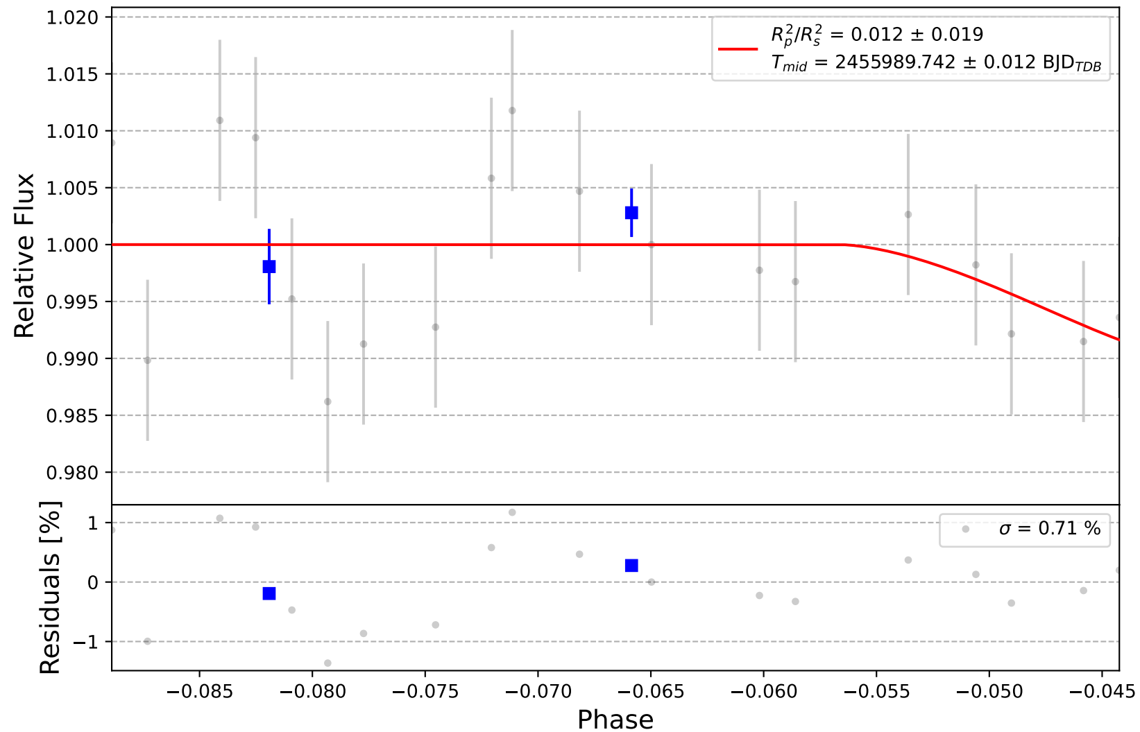
TrES-3 b
