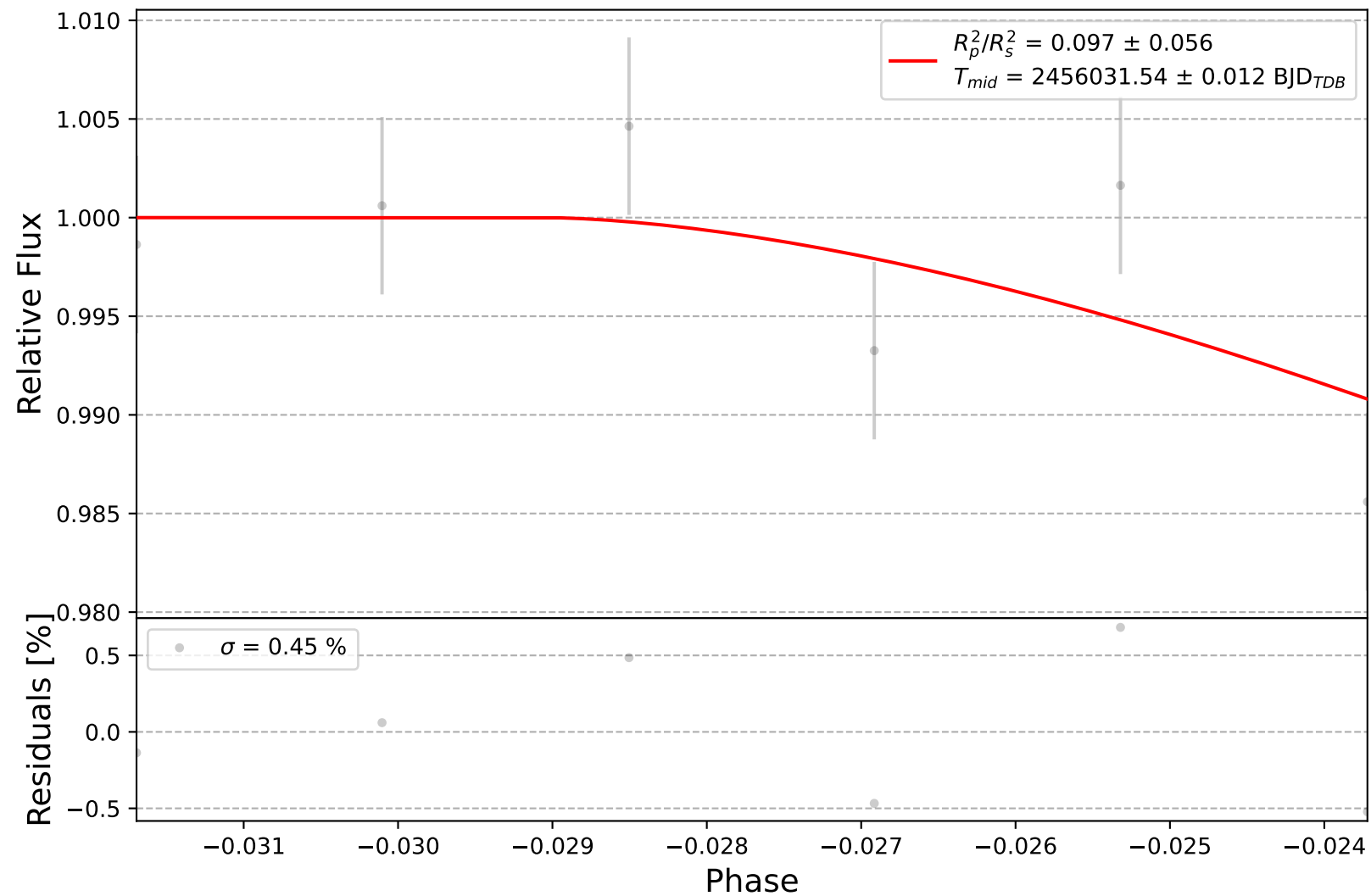
TrES-3 b
