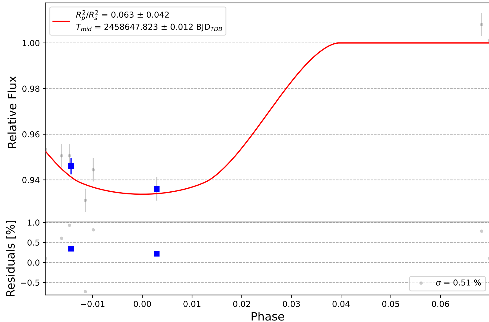
TrES-3 b
