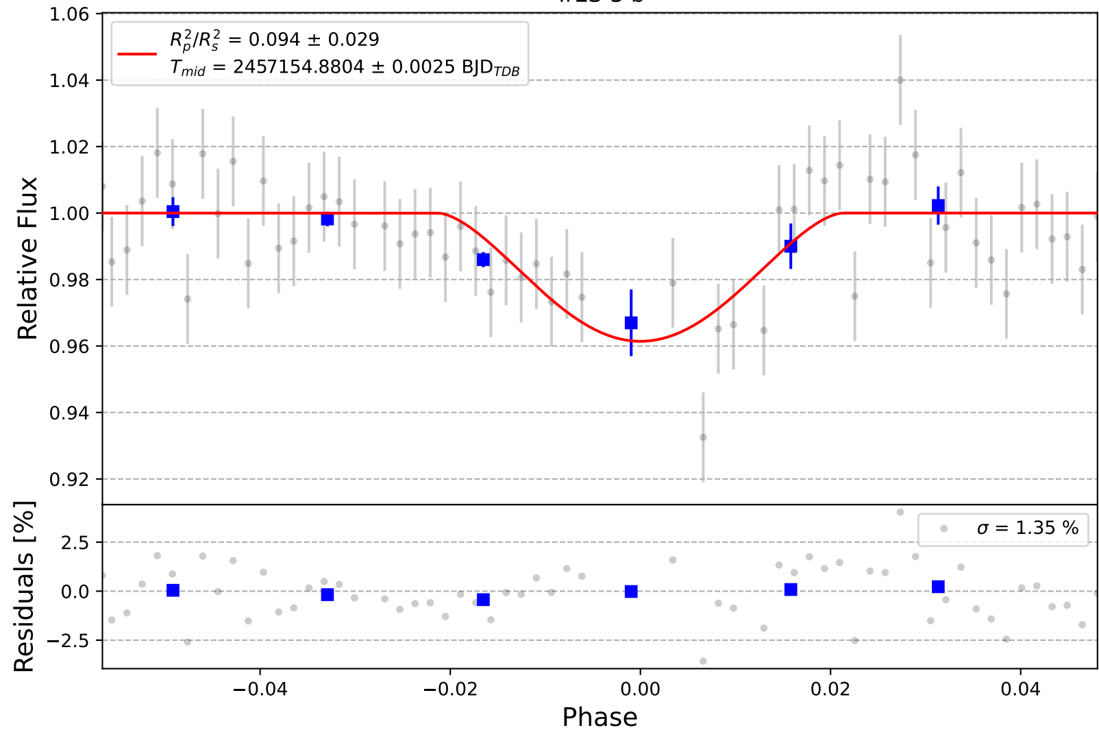
TrES-3 b
