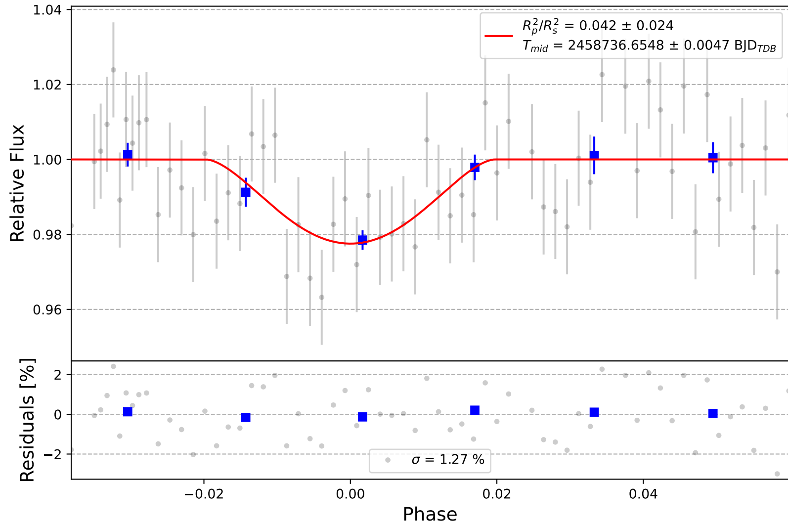
TrES-3 b
