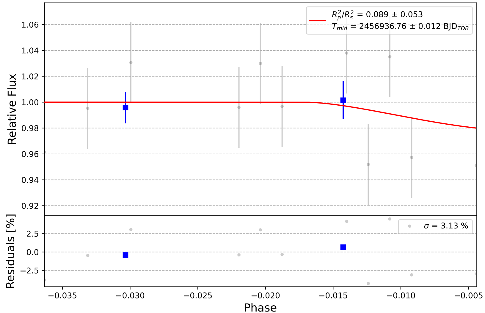
TrES-3 b
