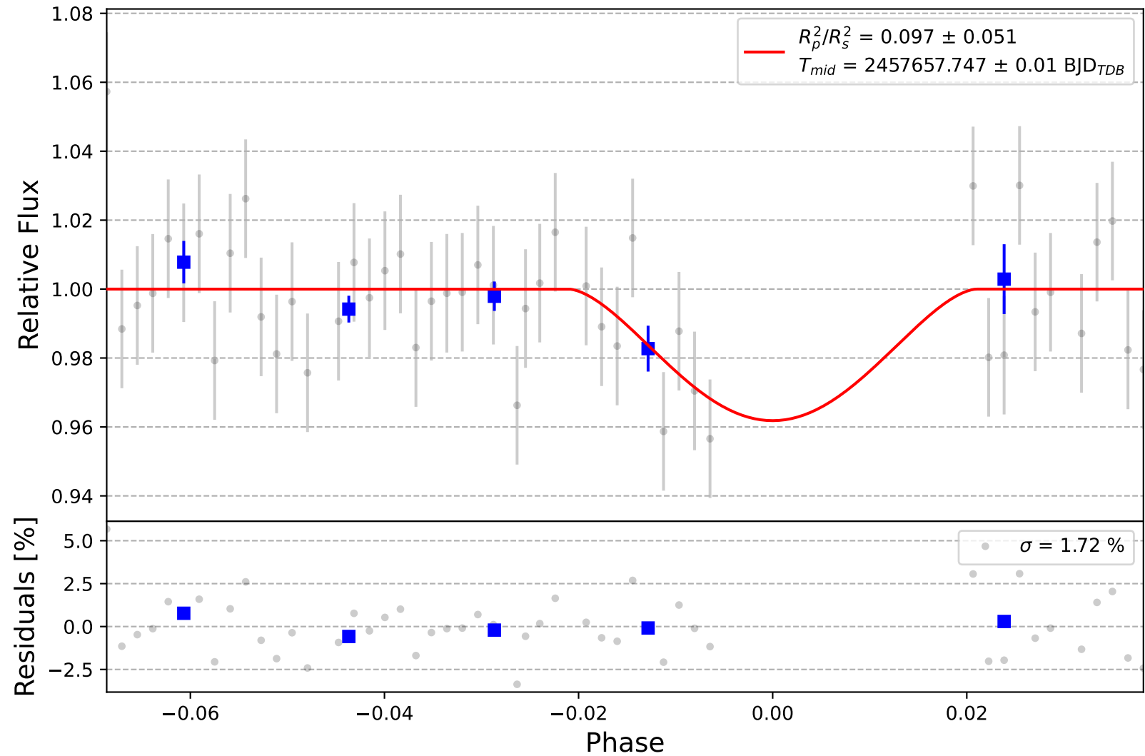
TrES-3 b
