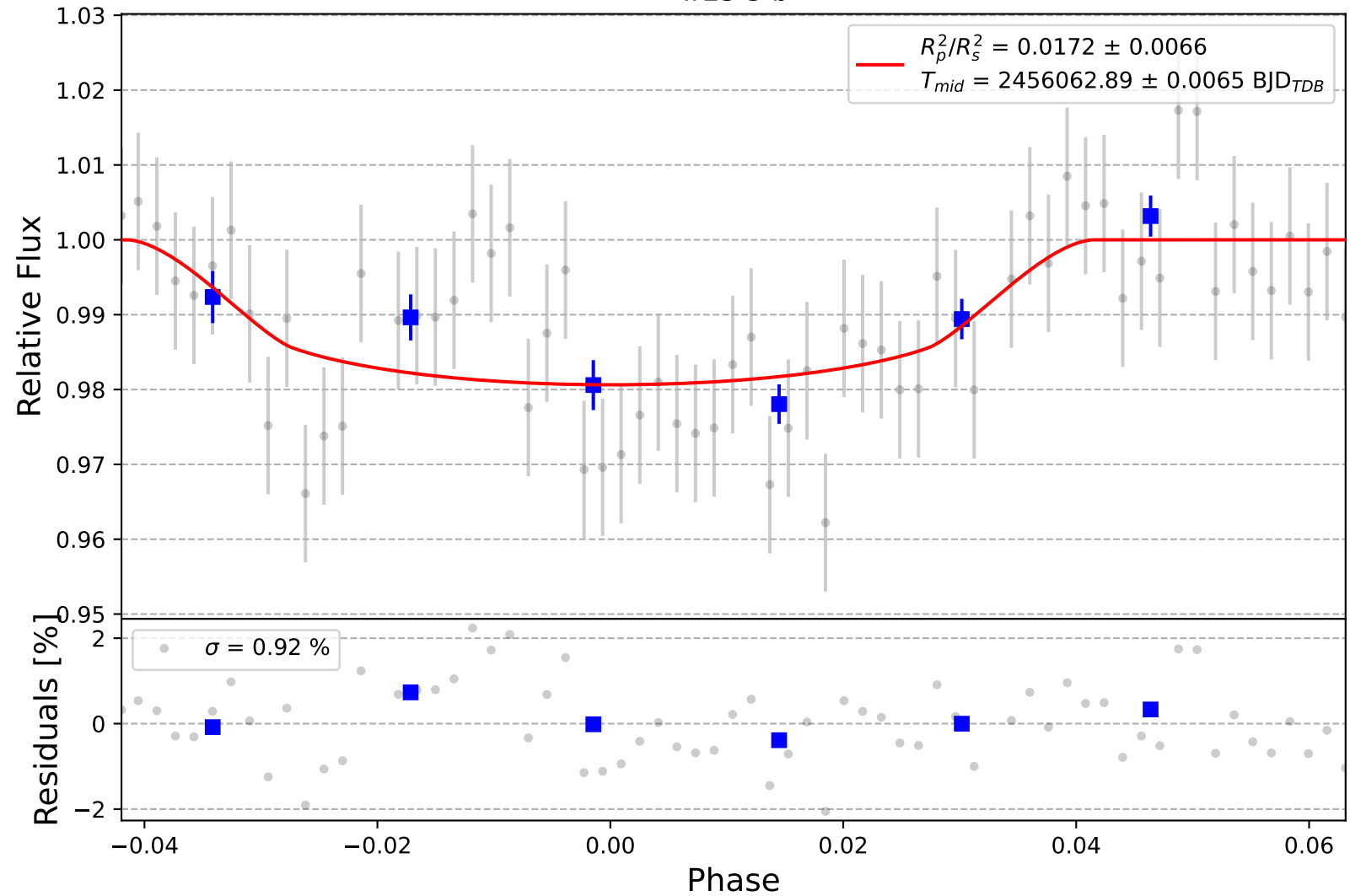
TrES-3 b
