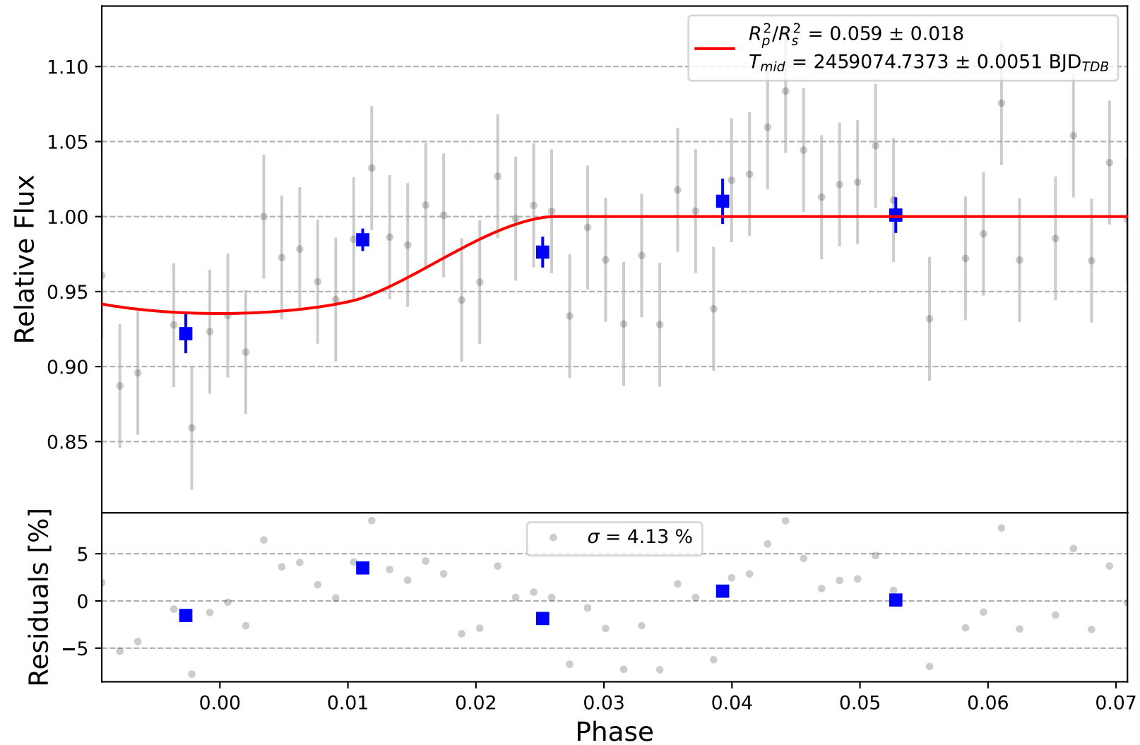
TrES-5 b
