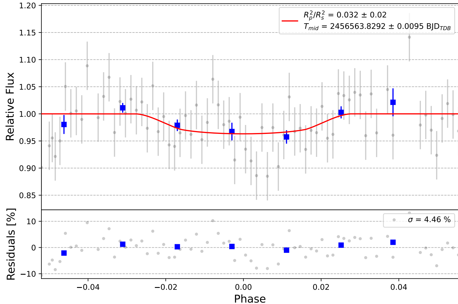
TrES-5 b
