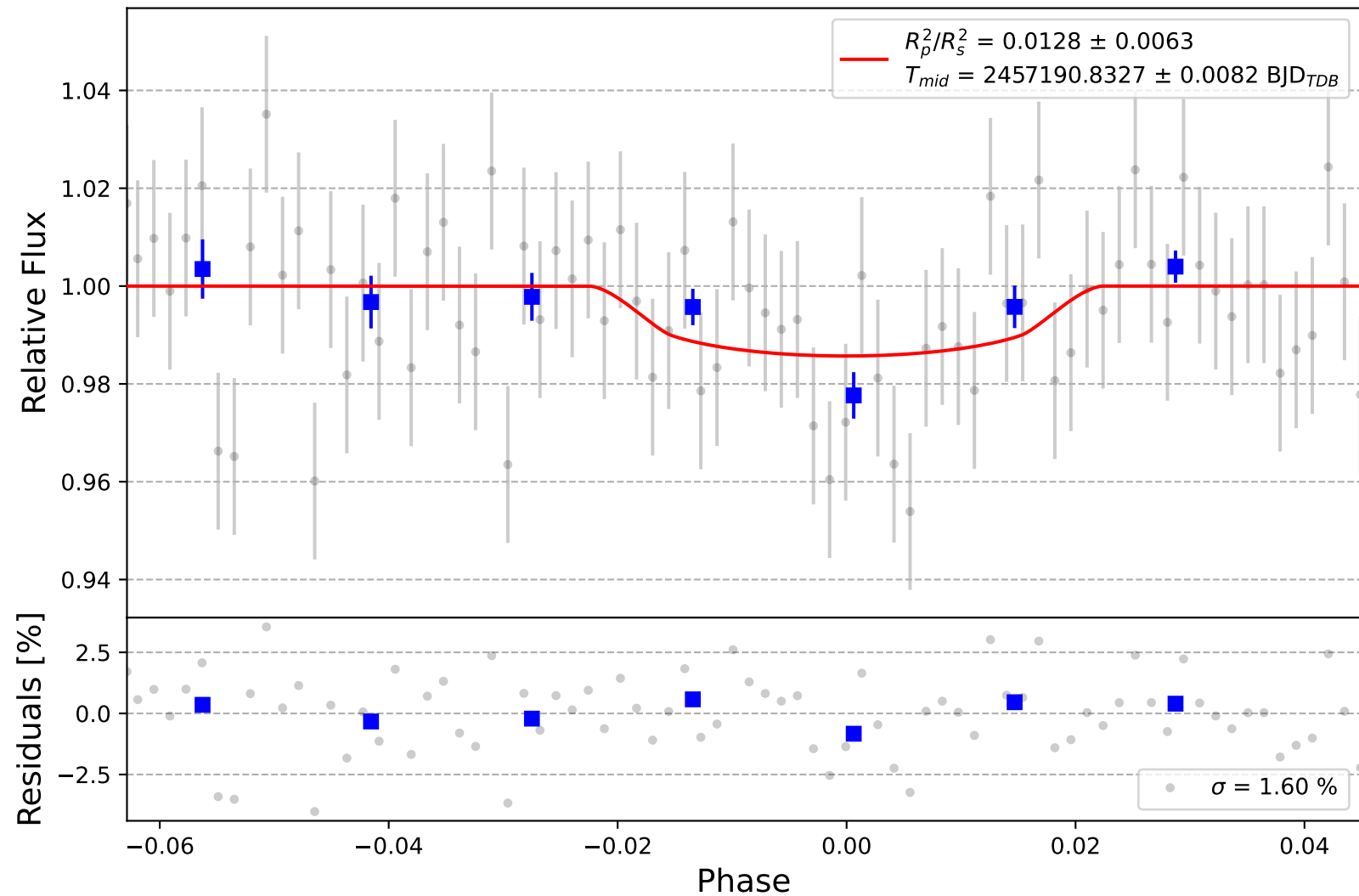
TrES-5 b
