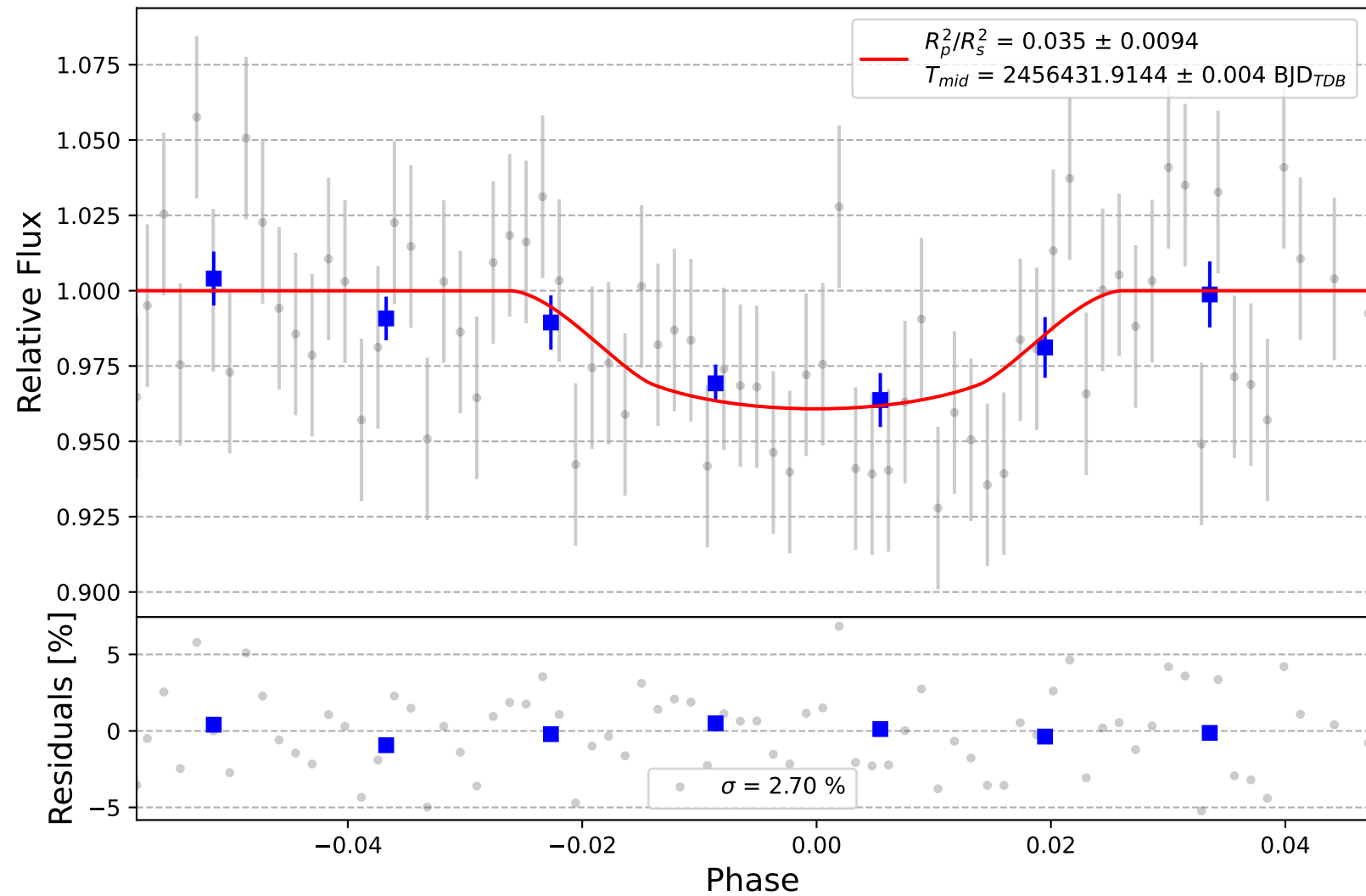
TrES-5 b
